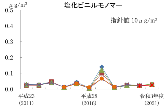
図 20 指針値設定物質の年平均値の経年変化
