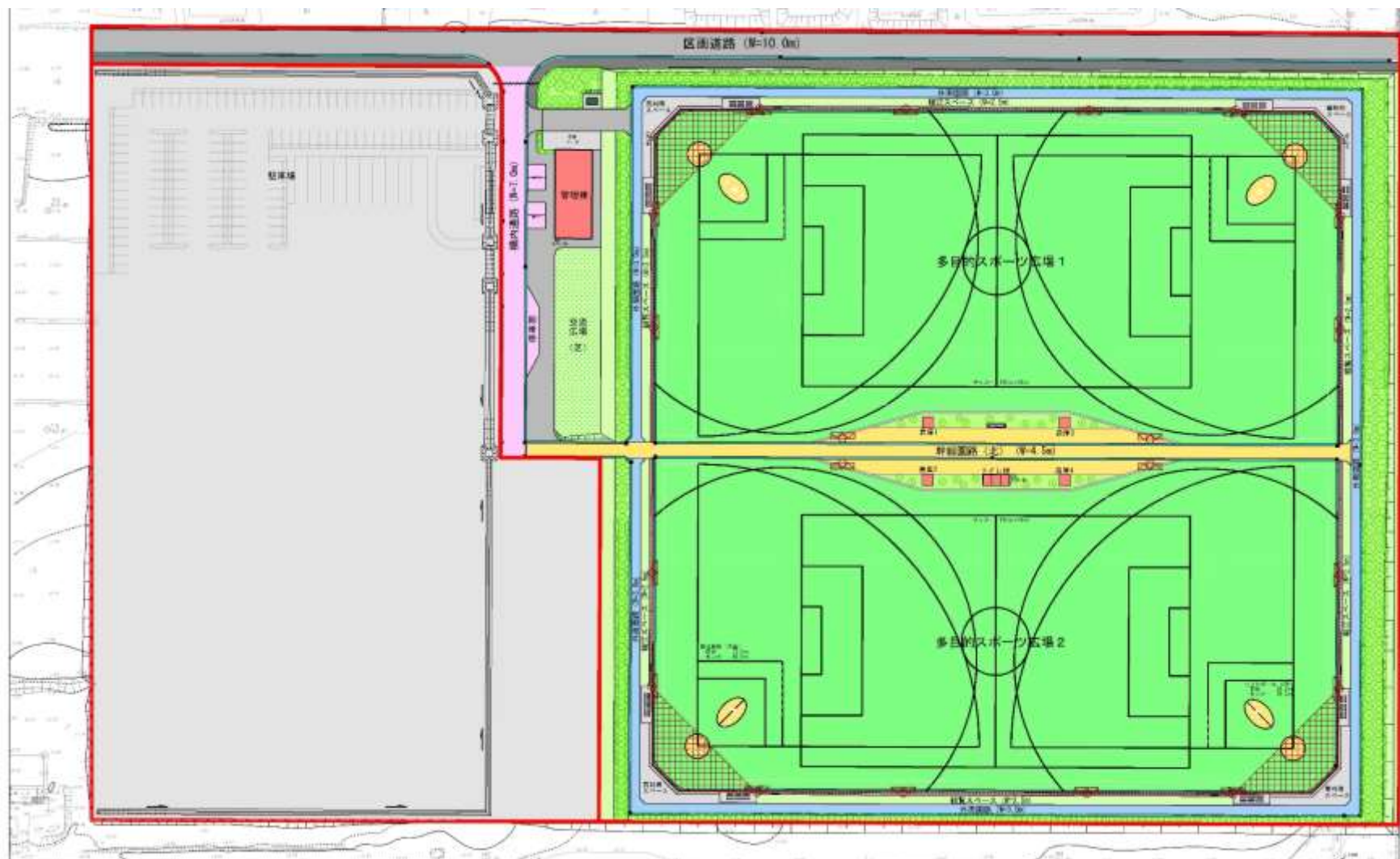
平面図（広島西飛行場跡地多目的スポーツ広場整備事業）
