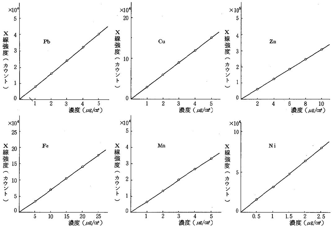
図3 検量線
