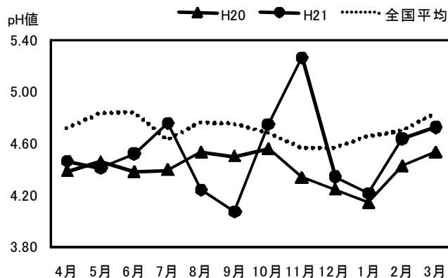
図 3 月別 pH 値及び全国平均値
