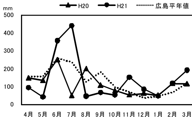
図 2 月別降水量及び平年値
