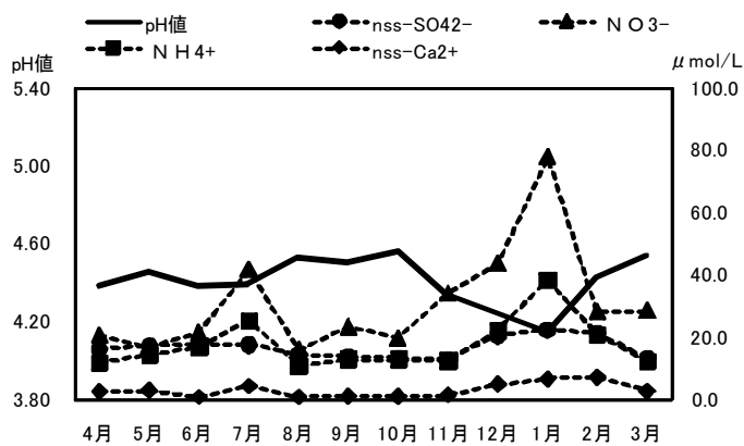
図 4-1 pH 値及び成分濃度(平成 20 年度)
