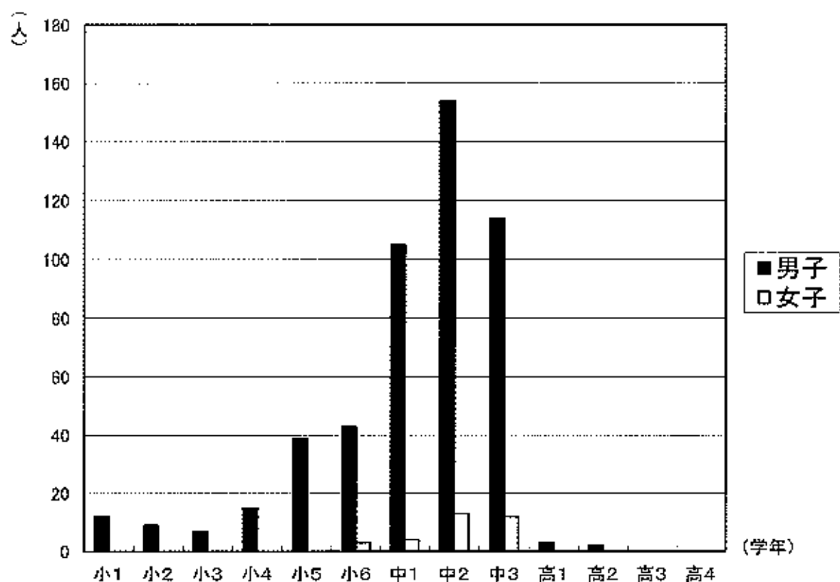
H25(実人数)
