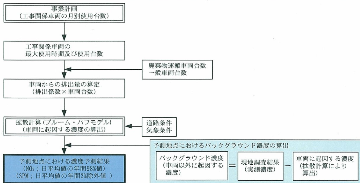
図 7-1.13 工事期間中の走行ルート沿道における NO 2 、SPM 濃度の予測手順
