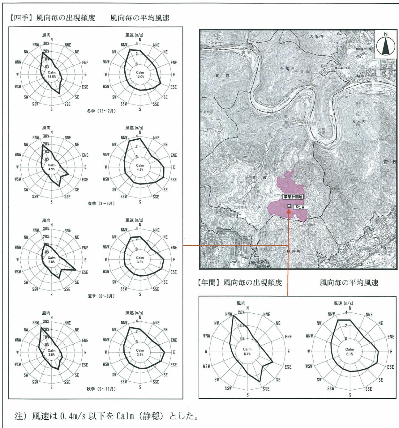
図 7-1.12 風向・風速調査結果(四季・年間)
