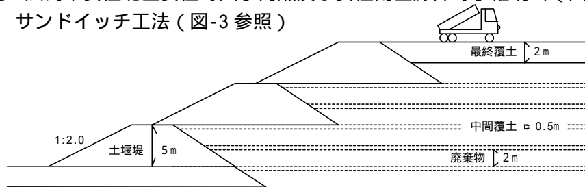
図-3 埋立方法 (サンドイッチ工法)
