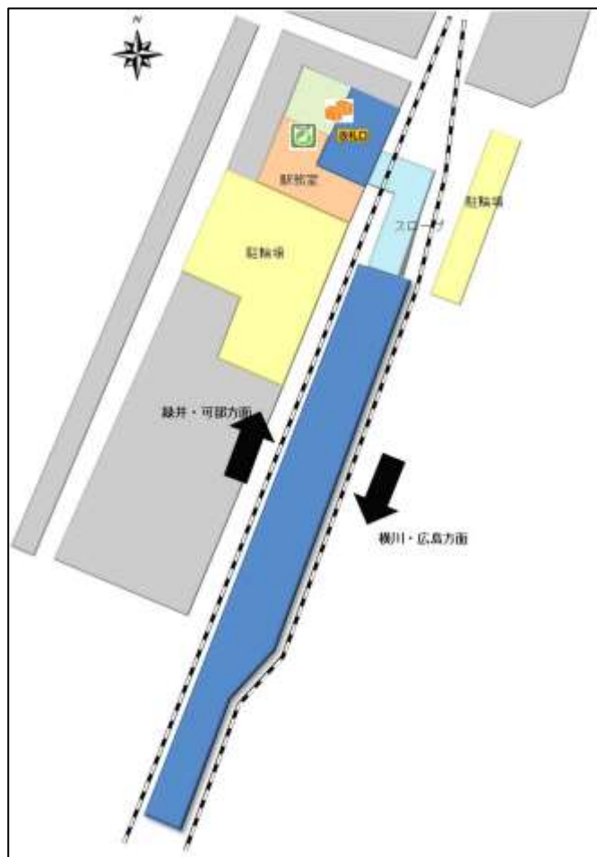
J R安芸長束駅 構内図
