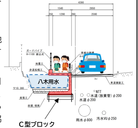
標準断面図 （安佐南1区125号線）
