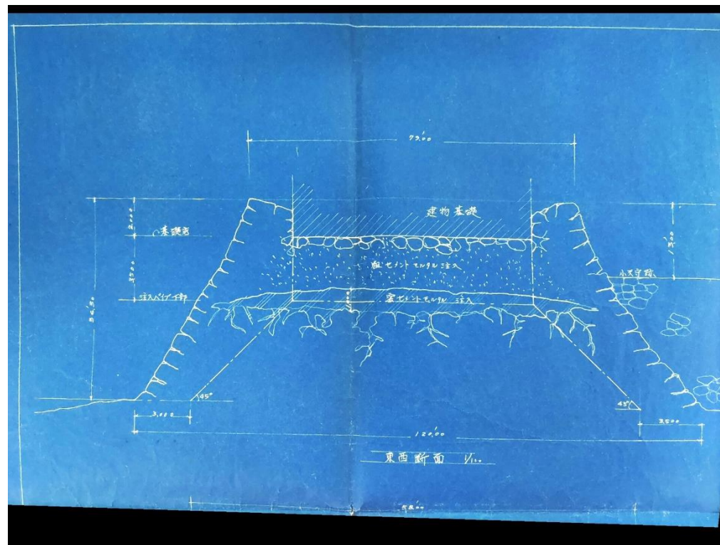
基礎グラウト図 広島城蔵
