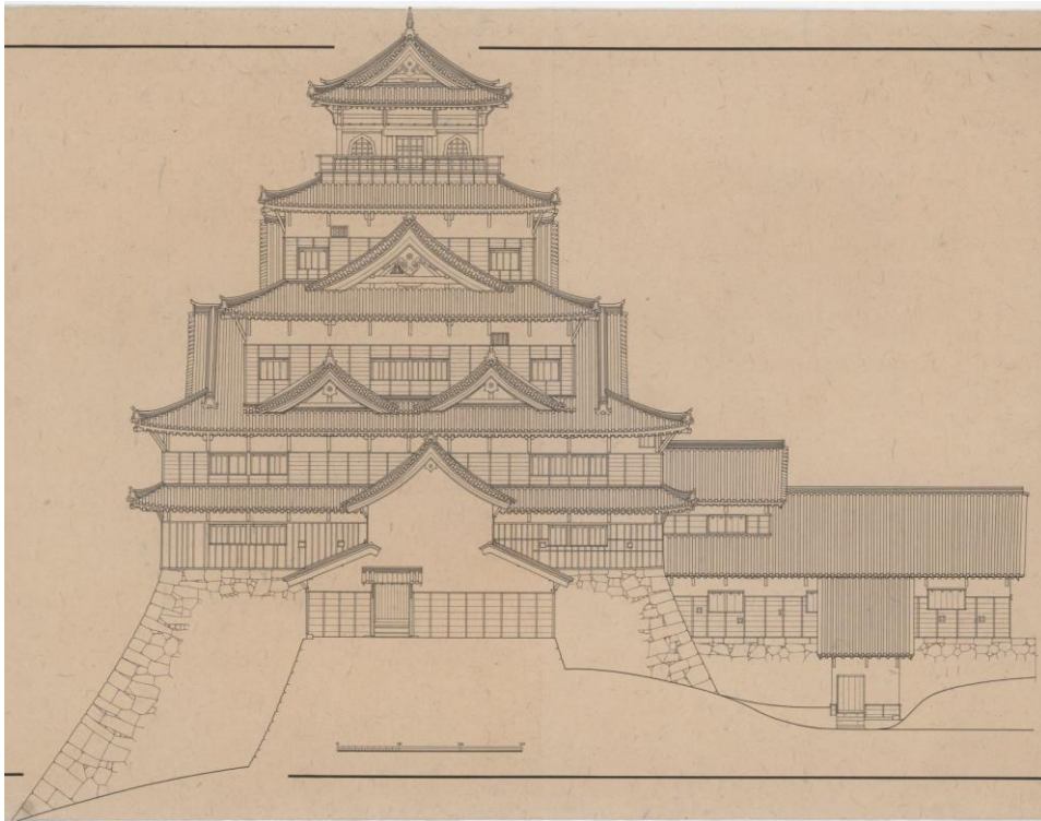
(左) 天守南立面図
