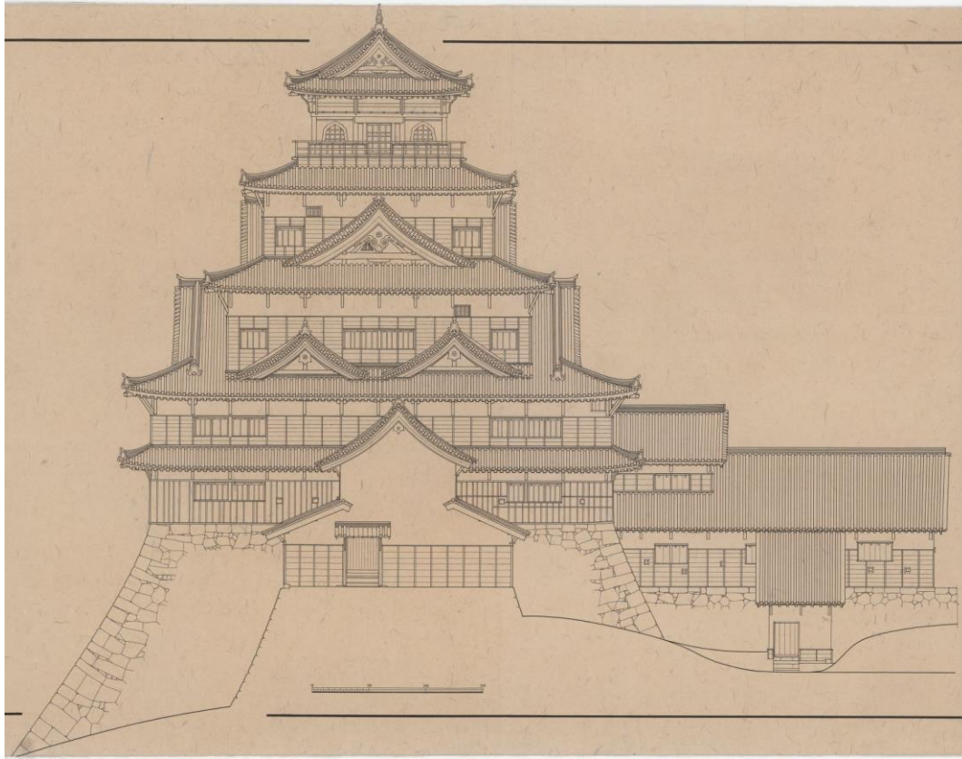
天守南立面図
