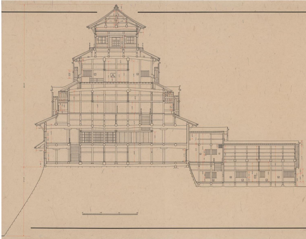
天守東西断面図
