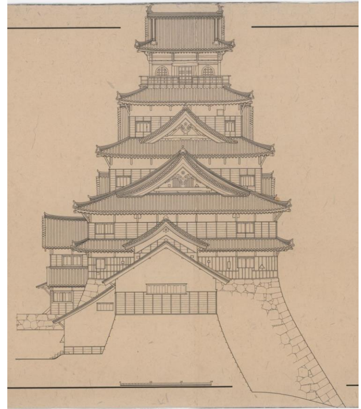
天守東立面図
