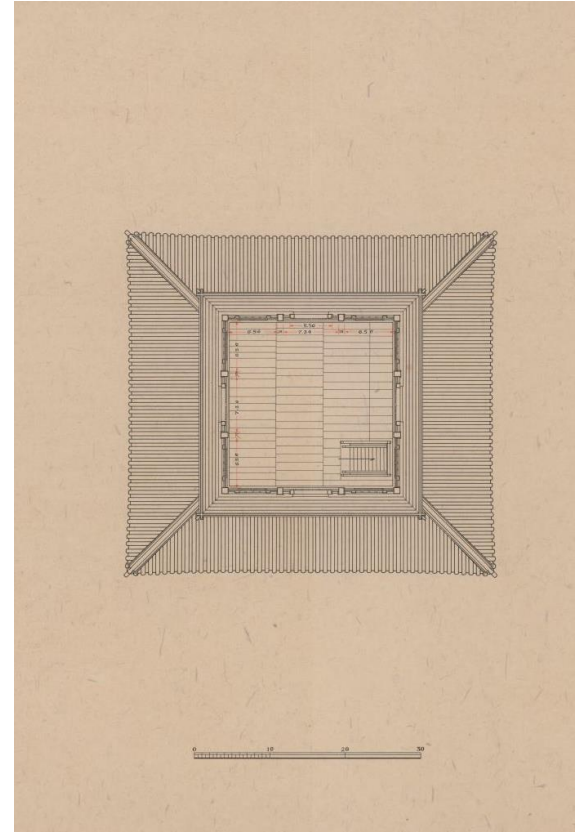
天守5階平面図
