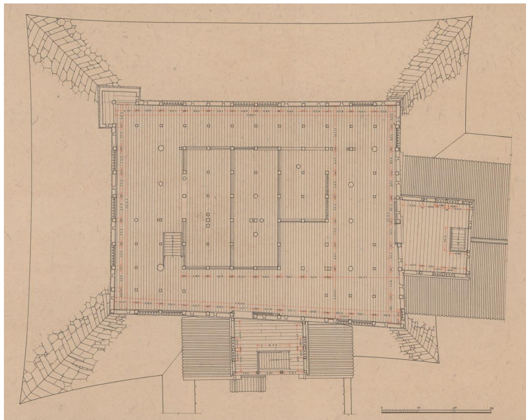
天守1階平面図及び南御廊下・東御廊下2階平面図
