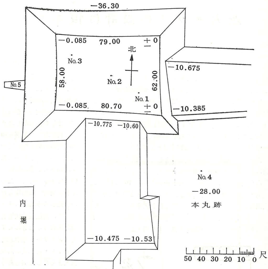
平図面 (ボーリング調査実施箇所No. 1~4)
