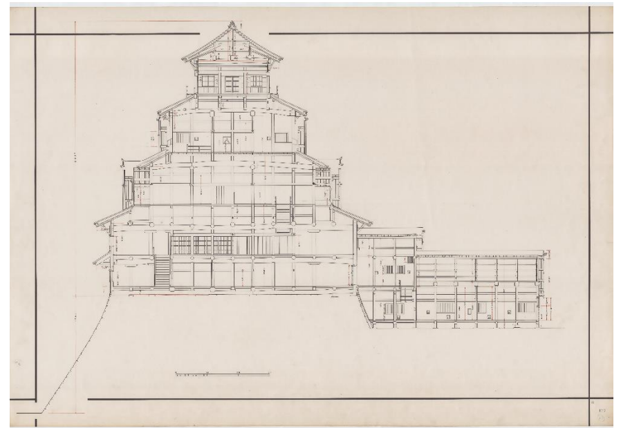
(右) 天守東西断面図
