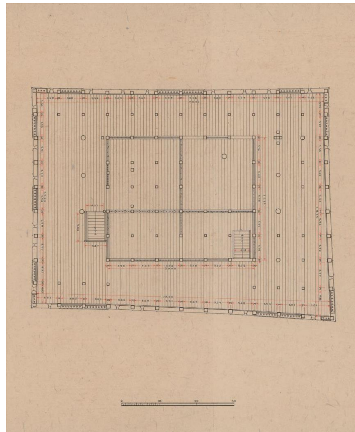
天守2階平面図
