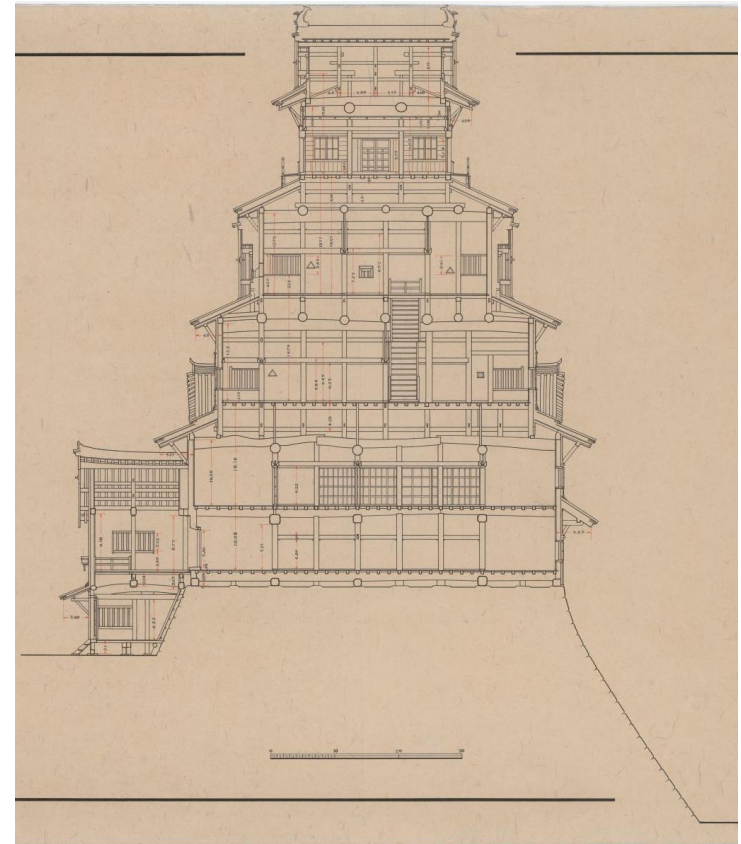
天守南北断面図
