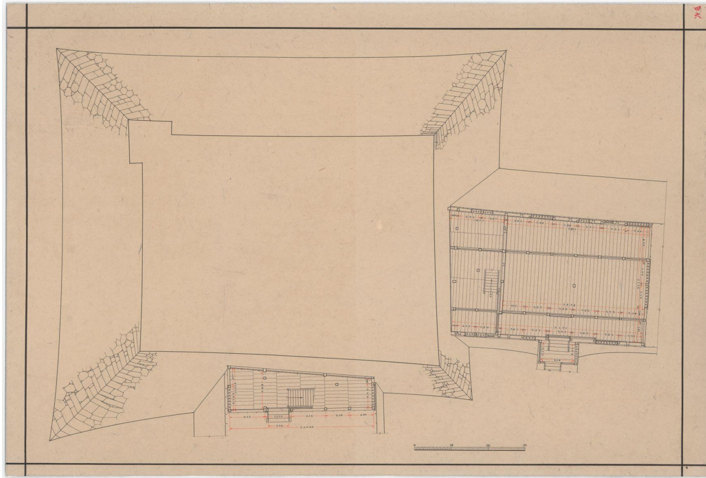
南御廊下・東御廊下1階平面図 姫路市立城郭研究室蔵
