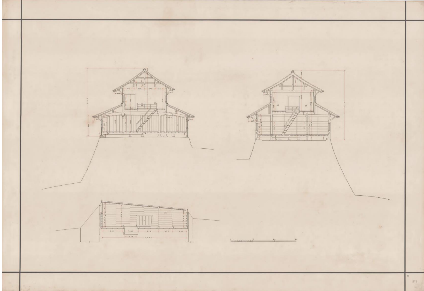
南御廊下断面図及び南御廊下1階平面図・東御廊下断面図 奈良文化財研究所蔵
