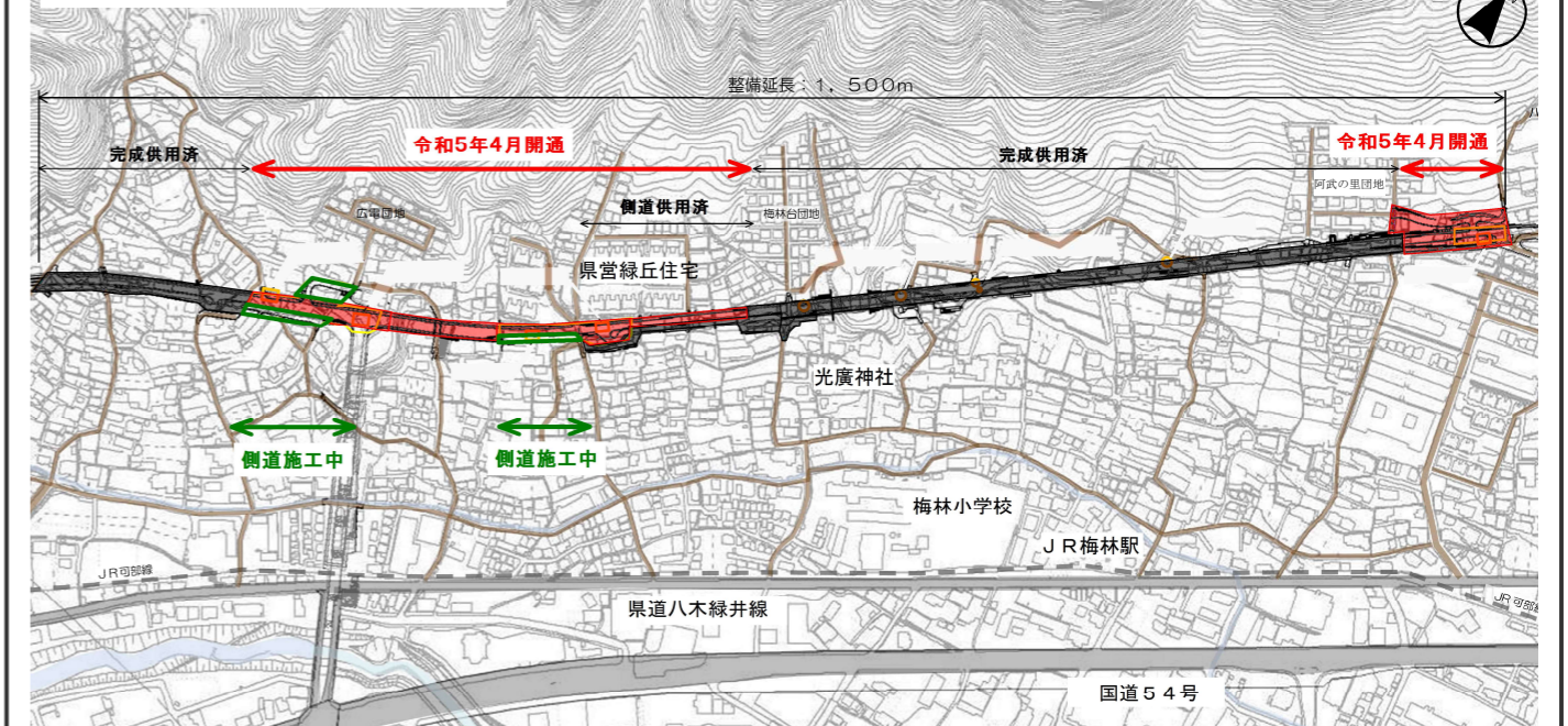
長束八木線（5工区）整備状況図
