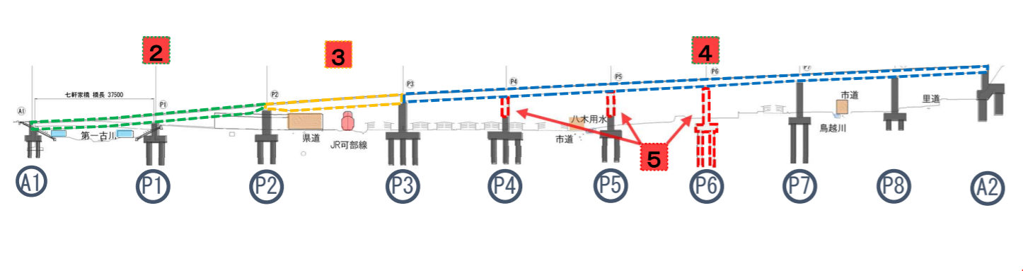
川の内線 縦断イメージ図
