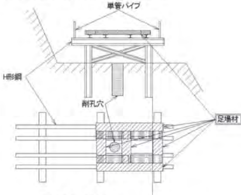
(C工法:作業采台概念図)
