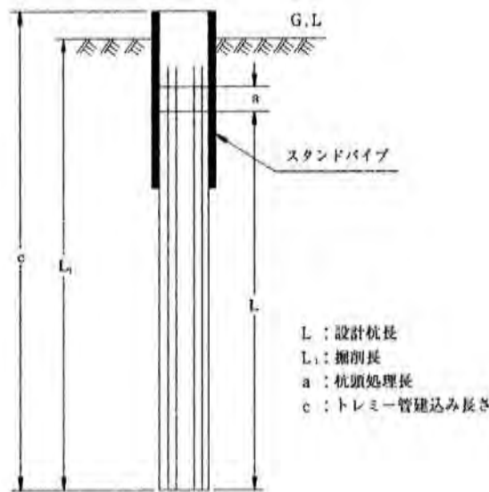
図 4-1 施工図
