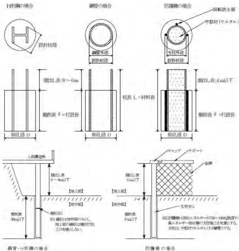
図 1-1 施工図
