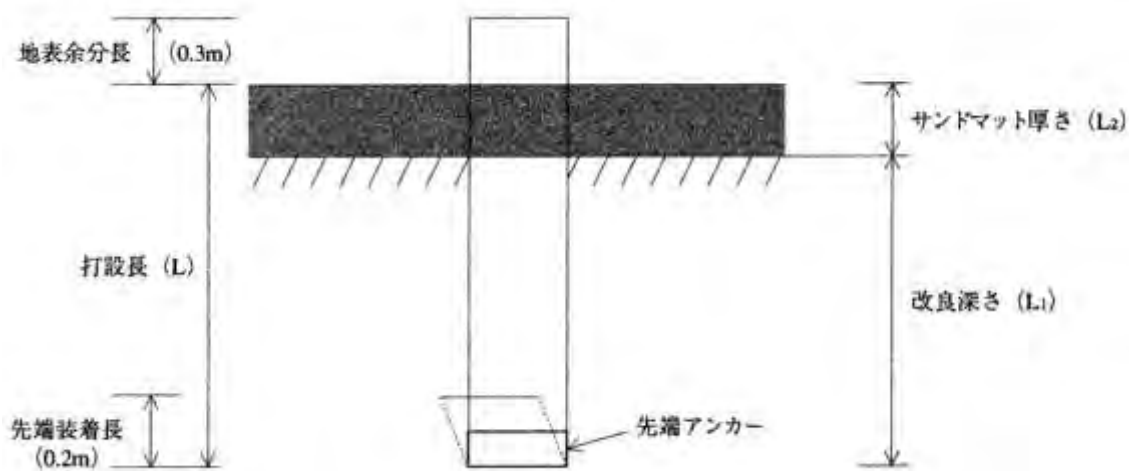
図 5.1 施工図
