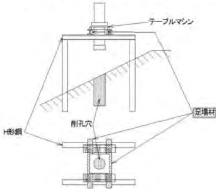
(C工法:作業采台概念図)
