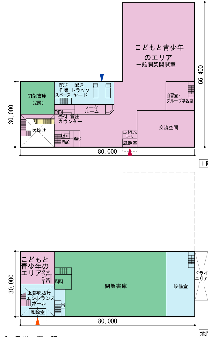
平面図
