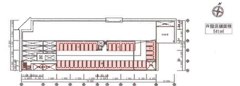
R階平面図 (R floor plan)
