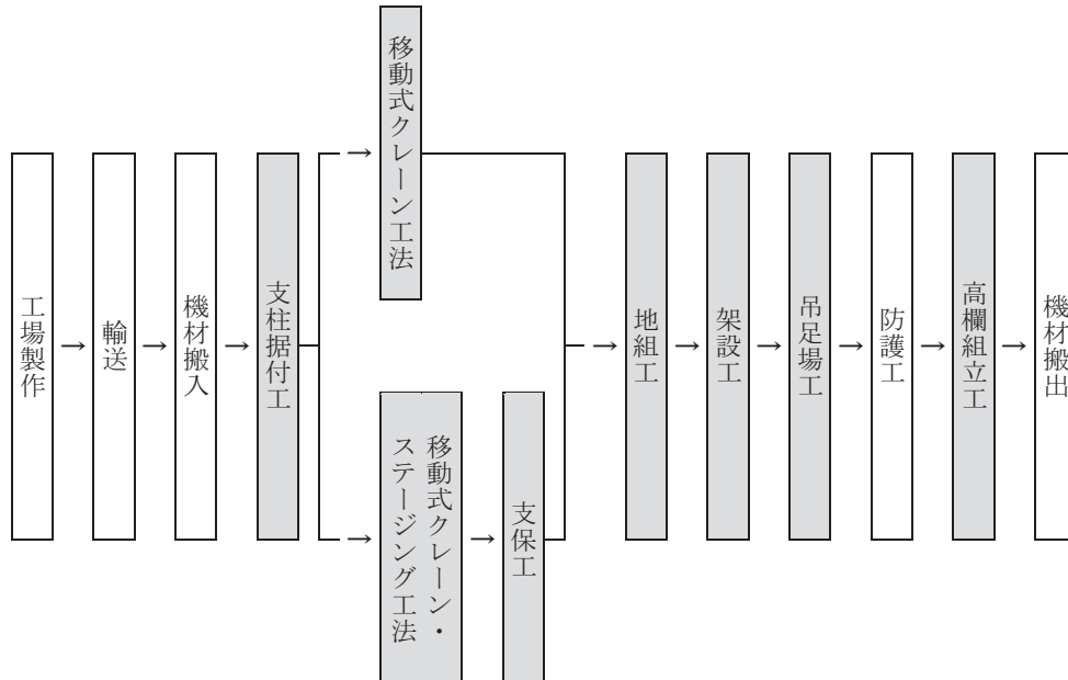
図 2-1 施工フロー
