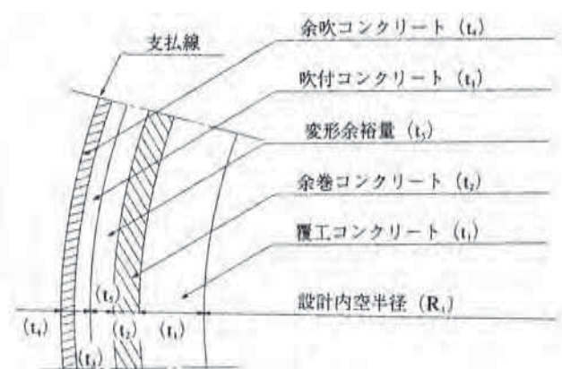
図 3.2 変形余裕を見込む場合
