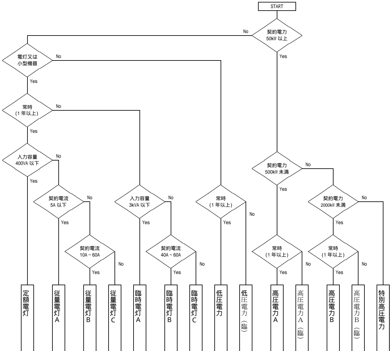
工事用電力の契約種別選定フロー
