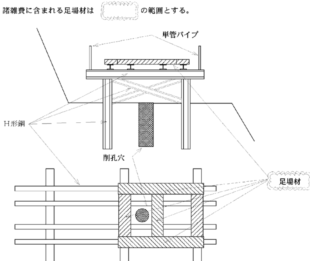
図 9-1 足場概念図
