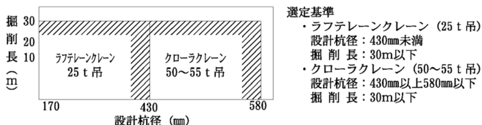
図 4-1 掘削用クレーン機種選定
