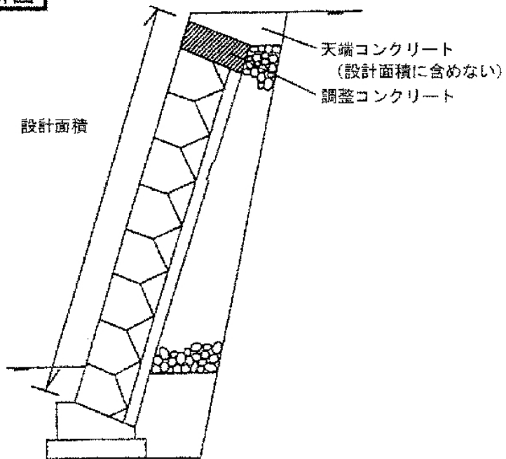
A-A断面
