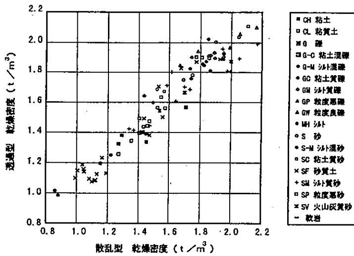
図一〇 散乱型と透過型の相関 (乾燥密度・土質別データ)
