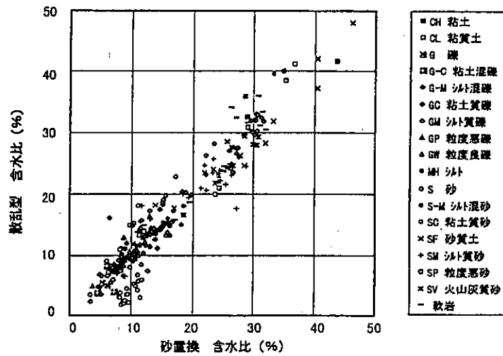
図一四 砂置換と散乱型の相関 (含水比・土質別データ)
