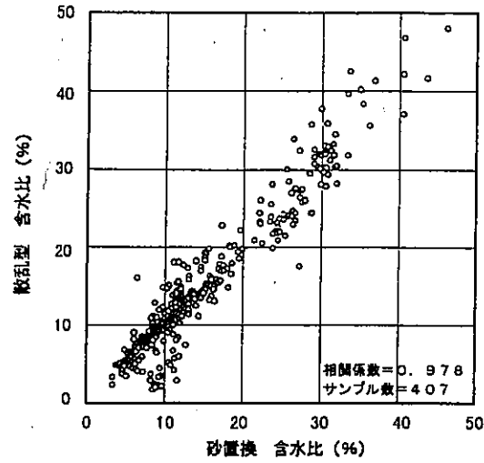
図一三 砂置換と散乱型の相関 (含水比・全データ)
