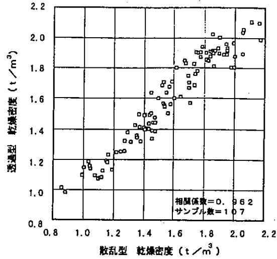
図一〇 散乱型と透過型の相関 (乾燥密度・全データ)
