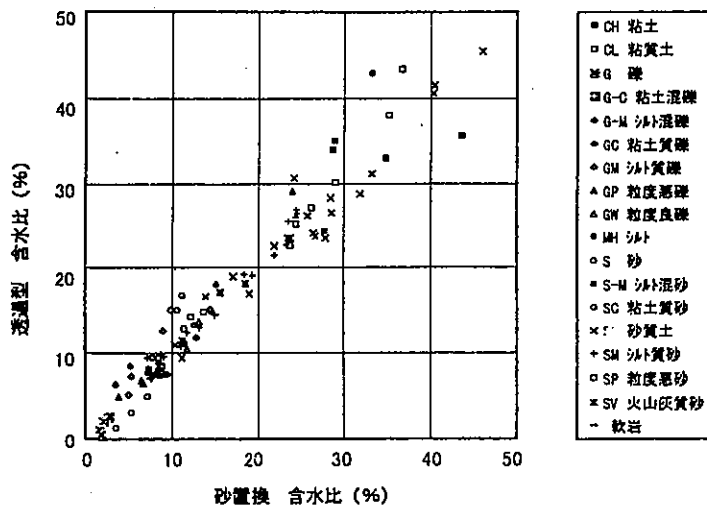
図一八 砂置換と透過型の相関 (含水比・土質別データ)
