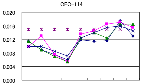
図3-1 CFC類調査地点別の経年変化
