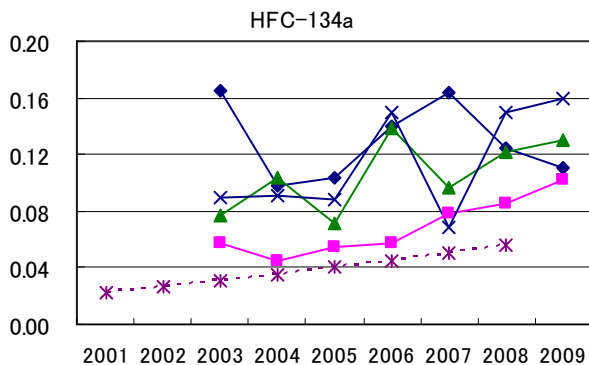
図 3-2 HCFC 類及び HFC の調査地点別経年変化
