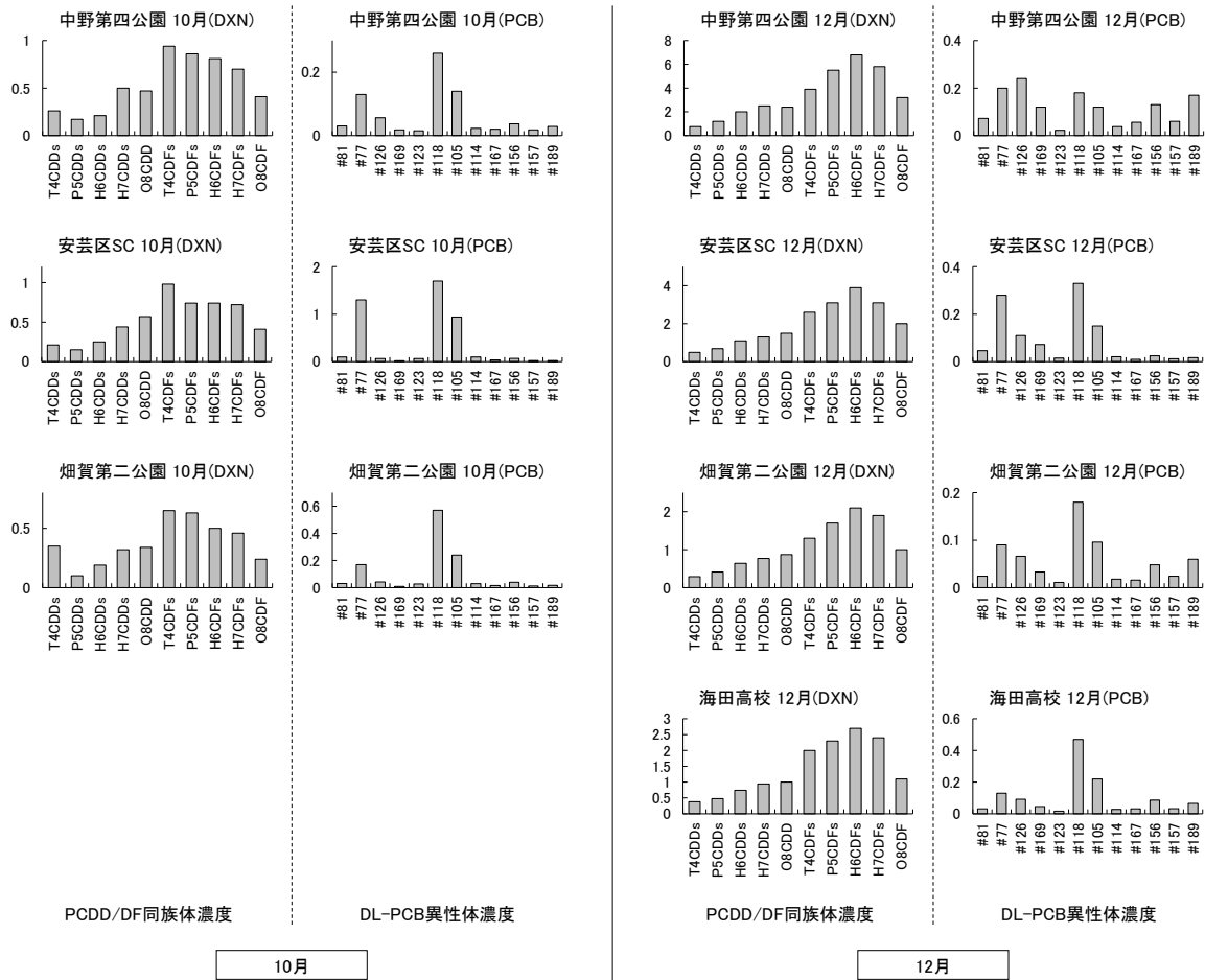
図8 同族体及び異性体のパターン
