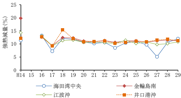
図5 底質(海域)の強熱減量
