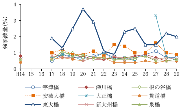
図4 底質(河川域)の強熱減量
