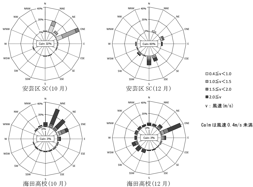
図9 風配図
