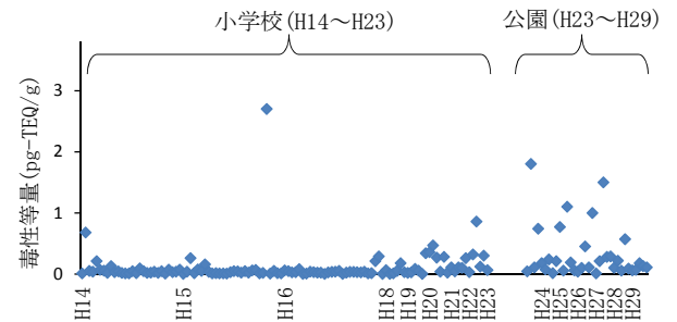
図6 土壌の用途別ダイオキシン類濃度
