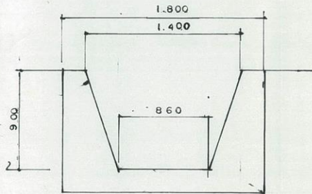
普通河川現況断面図
