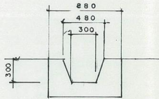
普通河川現況断面図
