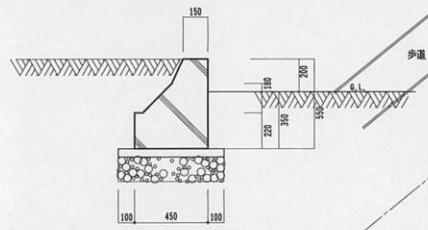
b-b' 擁壁断面図 1/30
