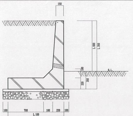
a-a' 擁壁断面図 1/30
