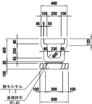
U型側溝 A1 S=1:20 A3 S=1:40 PU3-250
