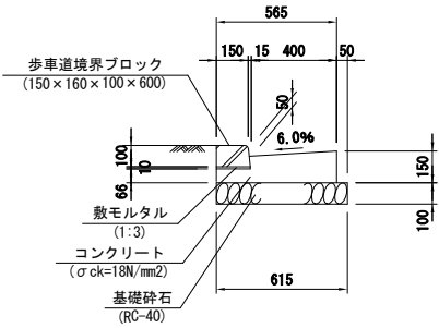
L型側溝 A1 S=1:20 A3 S=1:40
