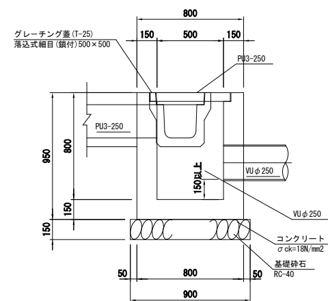
集水枋G1 A1 S=1:20 A3 S=1:40 G1-B500-L500-H800
