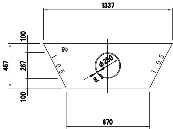
管渠 A1 S=1:20 A3 S=1:40 VU φ 250
