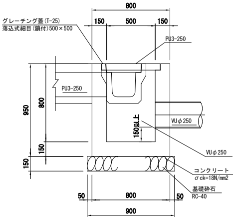
集水樹G1 A1 S=1:20 A3 S=1:40 G1-B500-L500-H800
