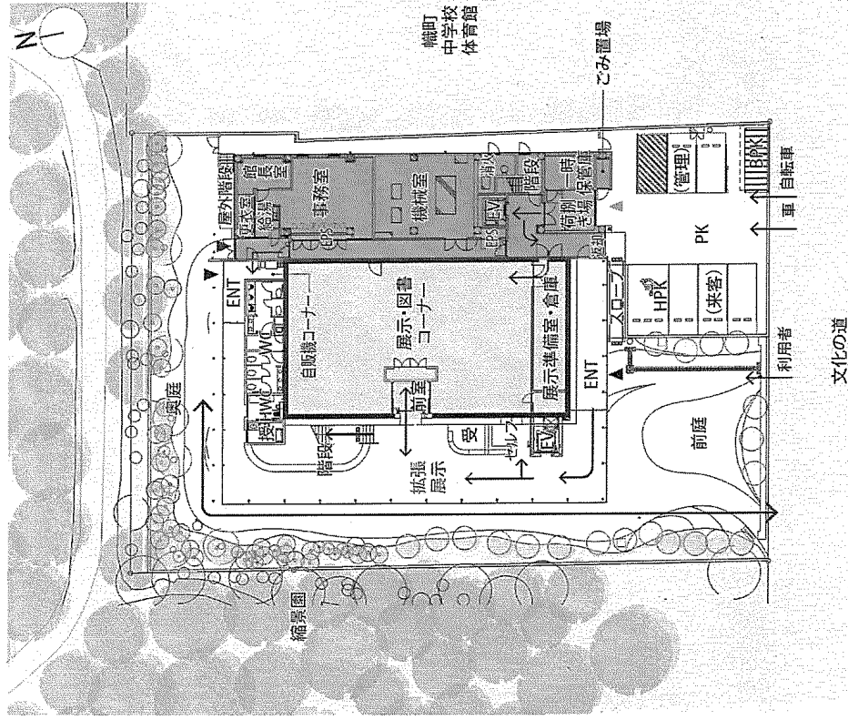
浅野文庫等施設（仮称）配置・平面計画
