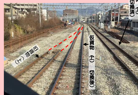
仮線路切り換え後（線路の接続が変わっています）
