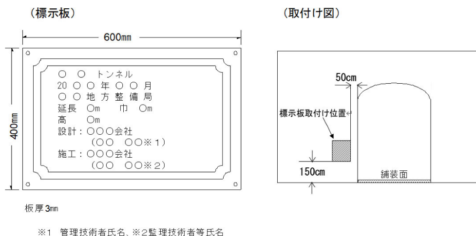
図 10-6-2 標示板の設置イメージ図
