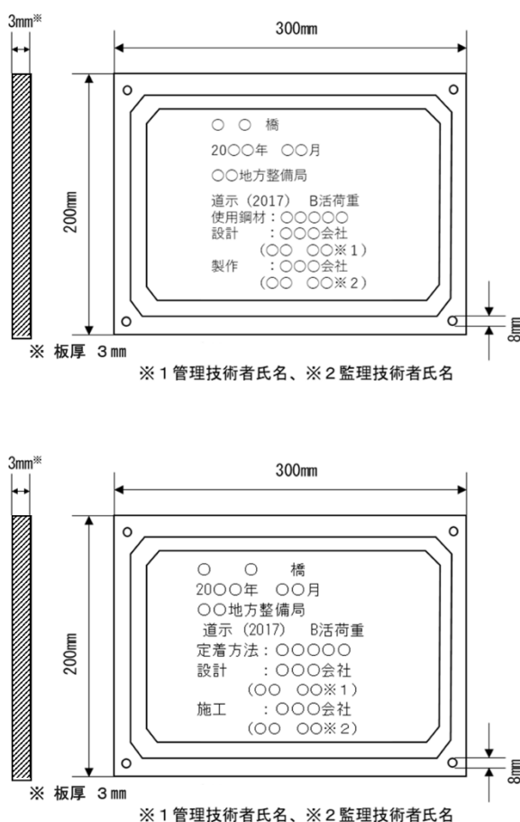
図 3-2-2 銘板の寸法及び記載事項
