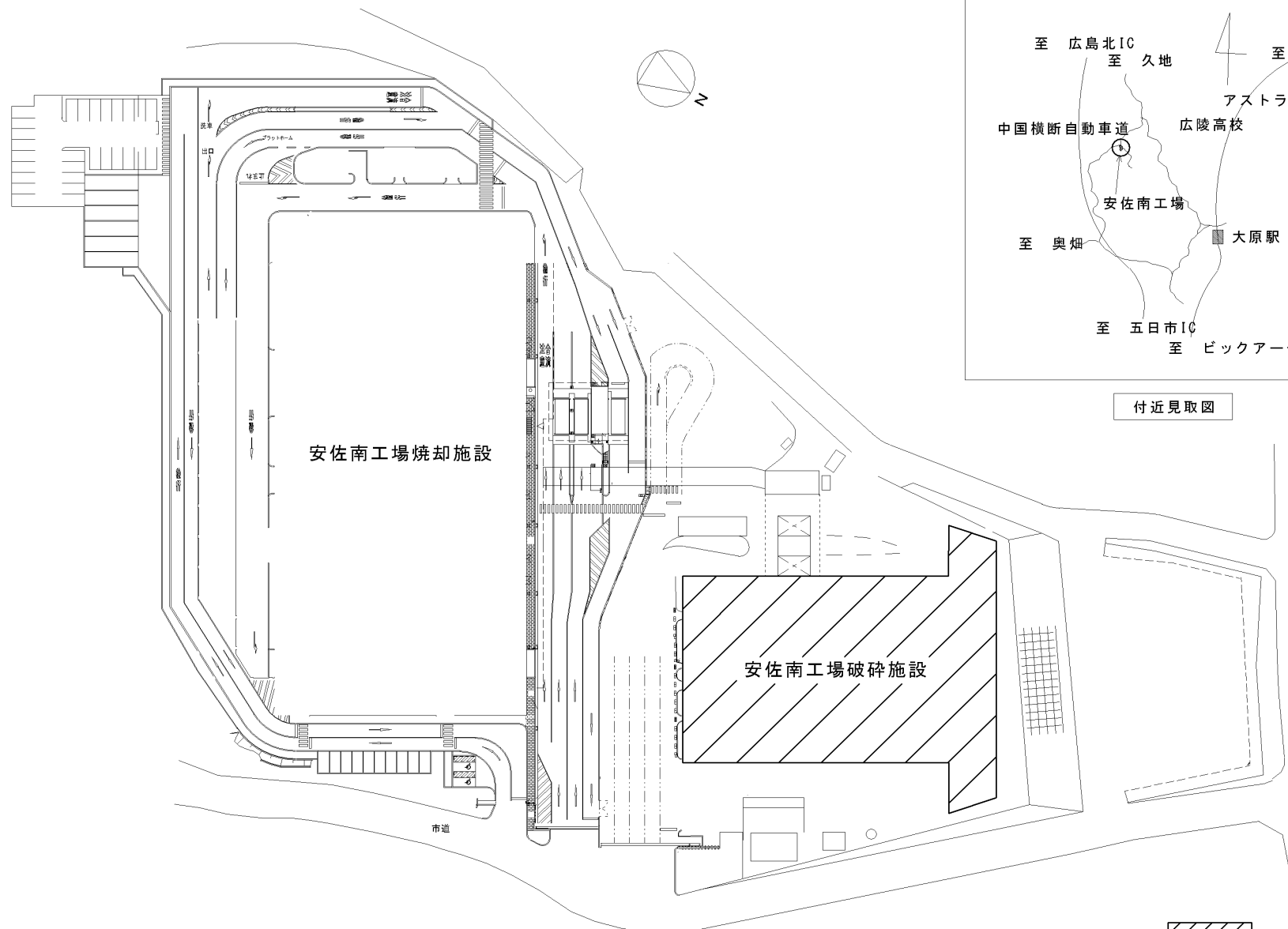
安佐南工場配置図
