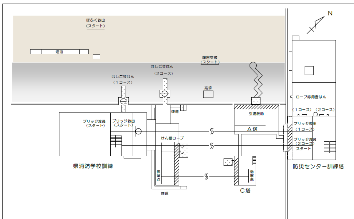
【別図6】施設図（陸上の部）
