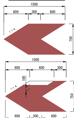
矢羽根型路面標示
