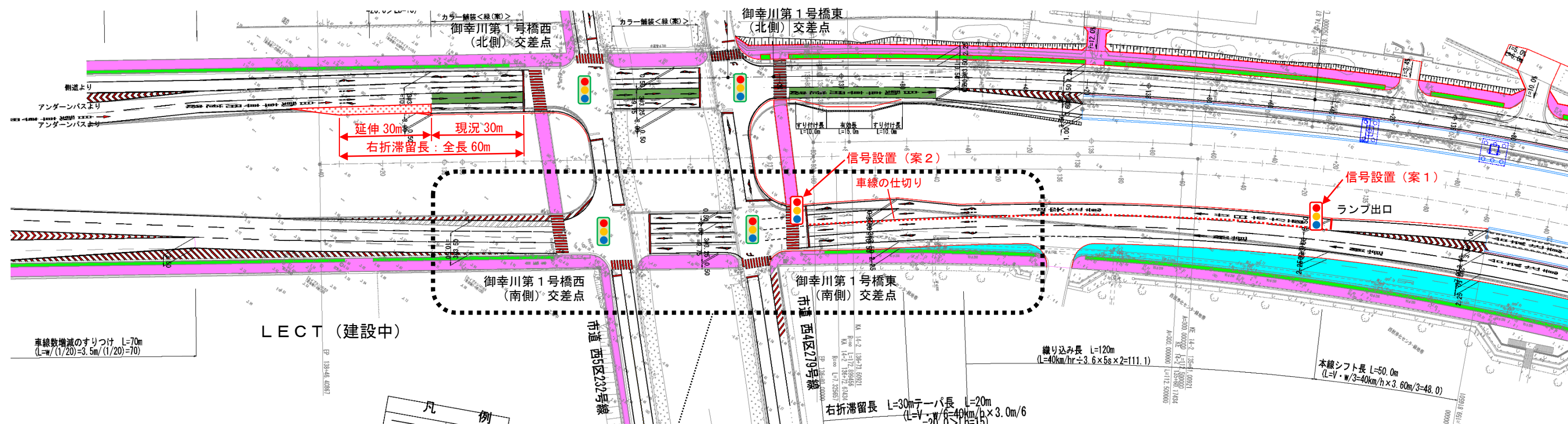
広島南道路の現況平面図
