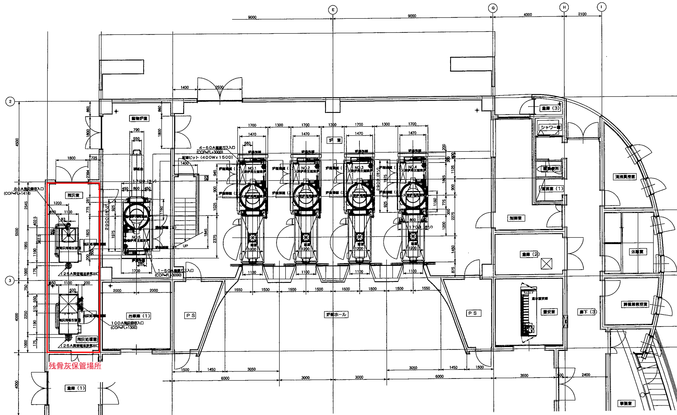
火葬炉1階平面配置図
