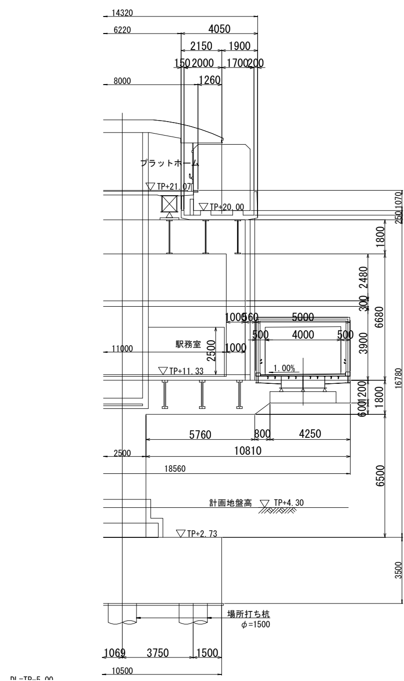
A - A' 断面図 (S=1/200)
