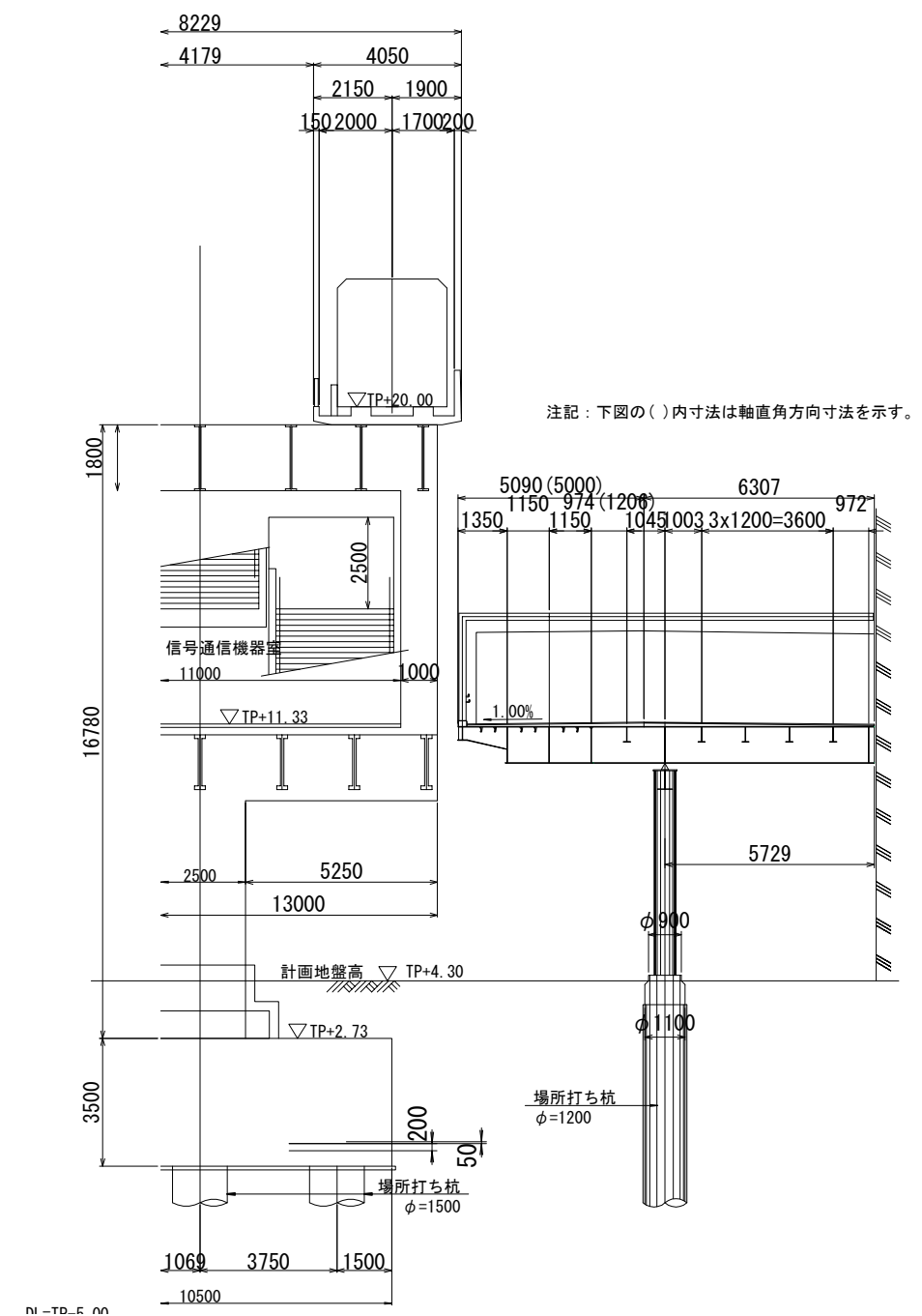
B - B' 断面图 (S=1/200)
