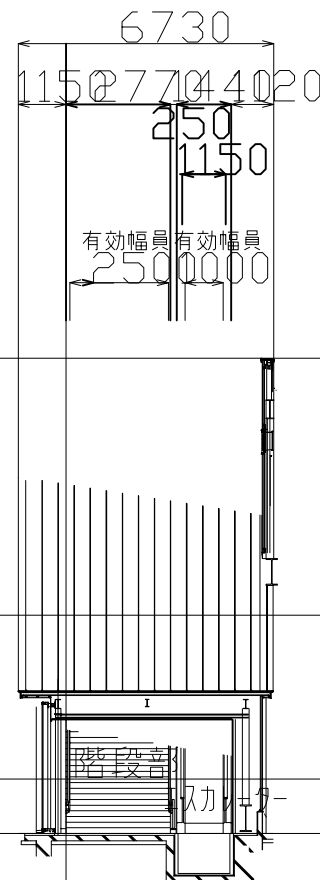
D - D' 断面図 (S=1/200)
