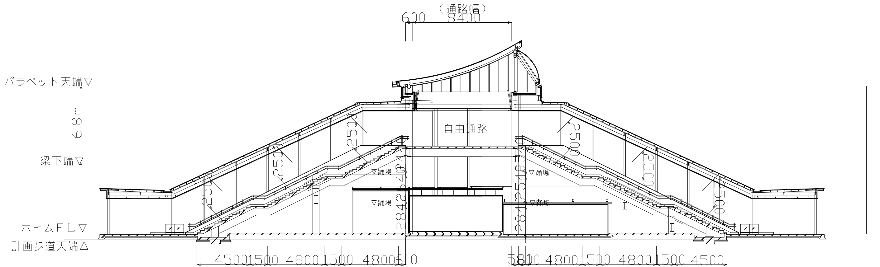
E - E' 断面図 (S=1/200)
