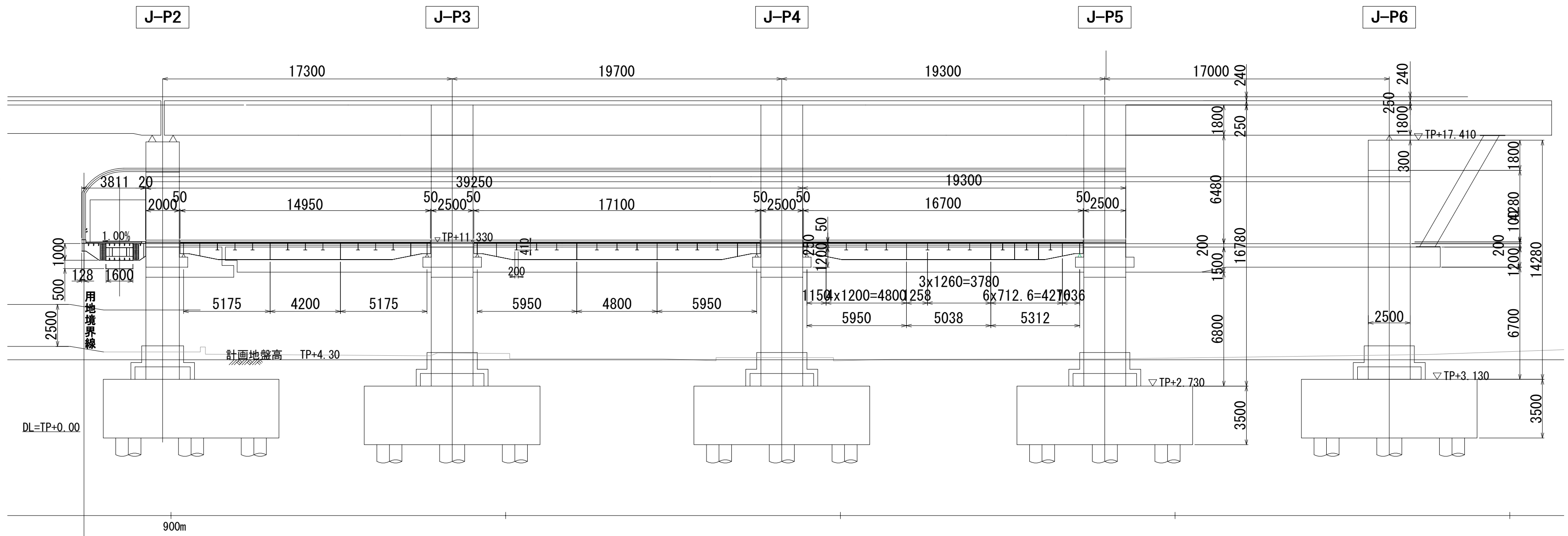
側面図 (S=1/200)
