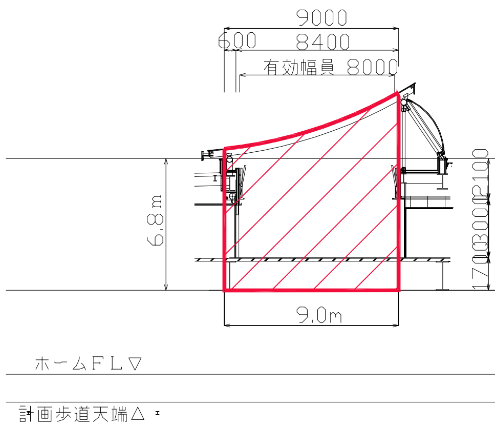
B - B' 断面図 (S=1/200)
