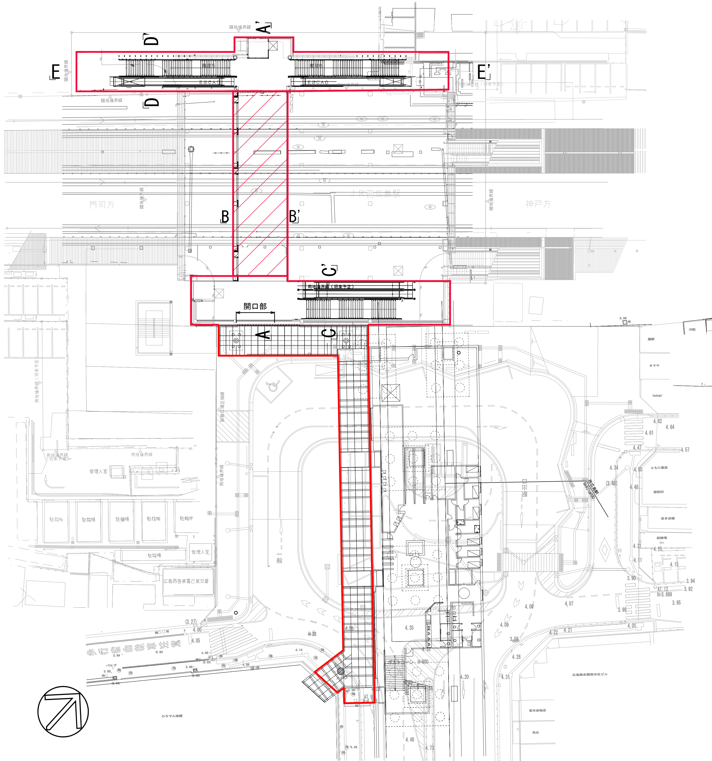
2F平面図 (S=1/300)
