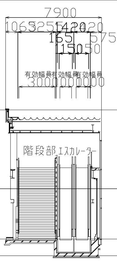
C - C' 断面図 (S=1/200)
