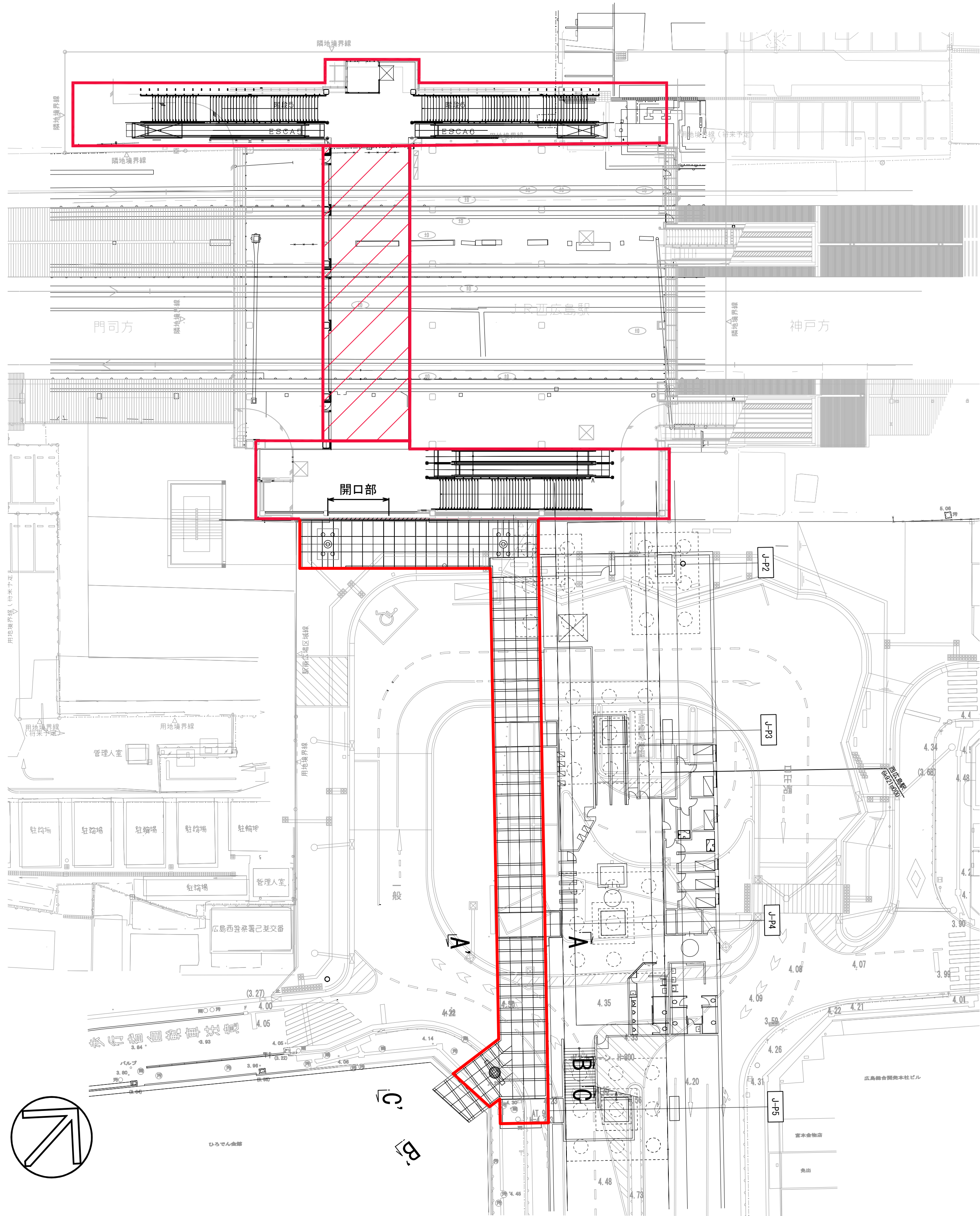
2F平面図 (S=1/300)
