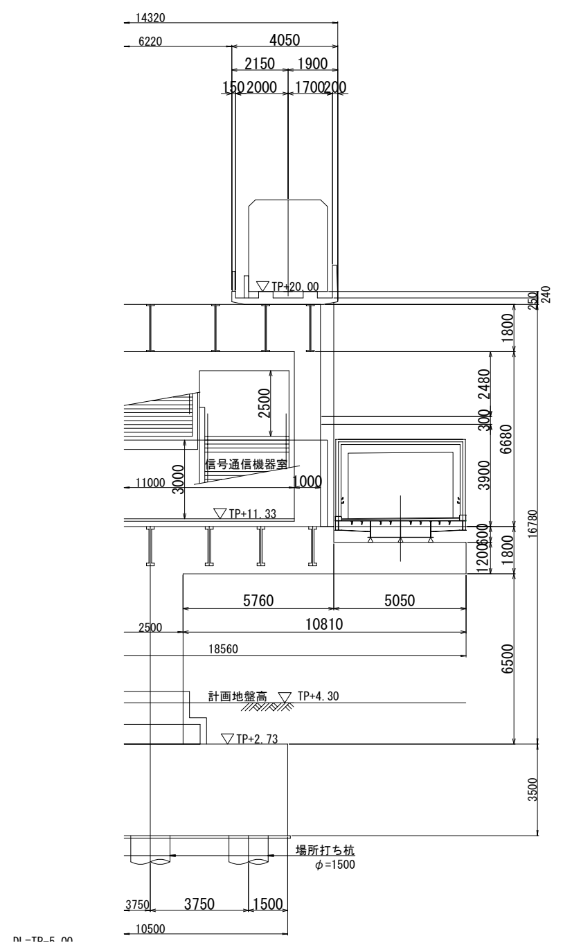
C - C' 断面图 (S=1/200)
