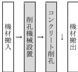
図 2-1 施工フロー
