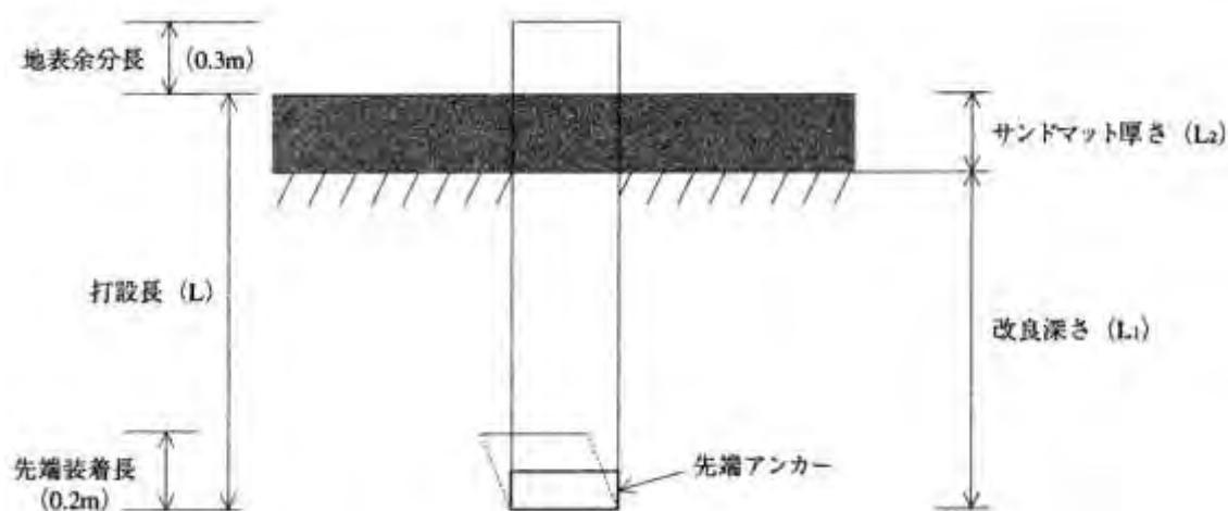
図 5.1 施工図
