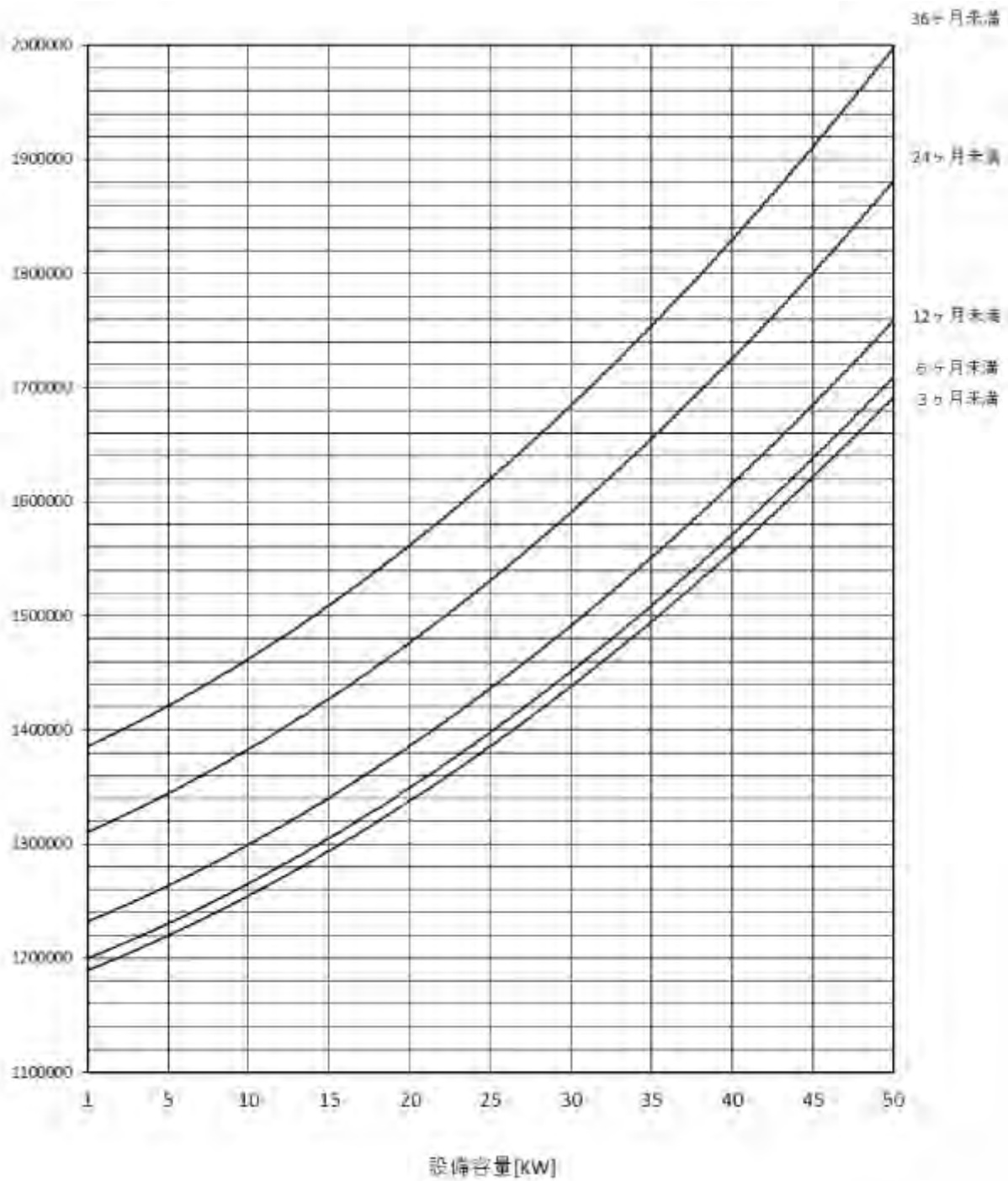
グラフ-(1) 土木工事仮設用電力設備費積算グラフ[低圧受電設備]
