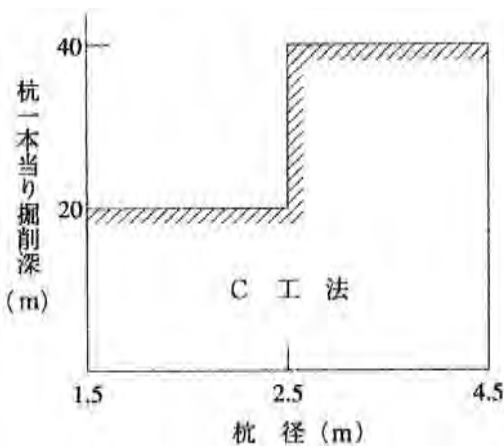
図 1-2 適用杭径及び掘削深（掘削機が現場に搬入出来ない場合）
