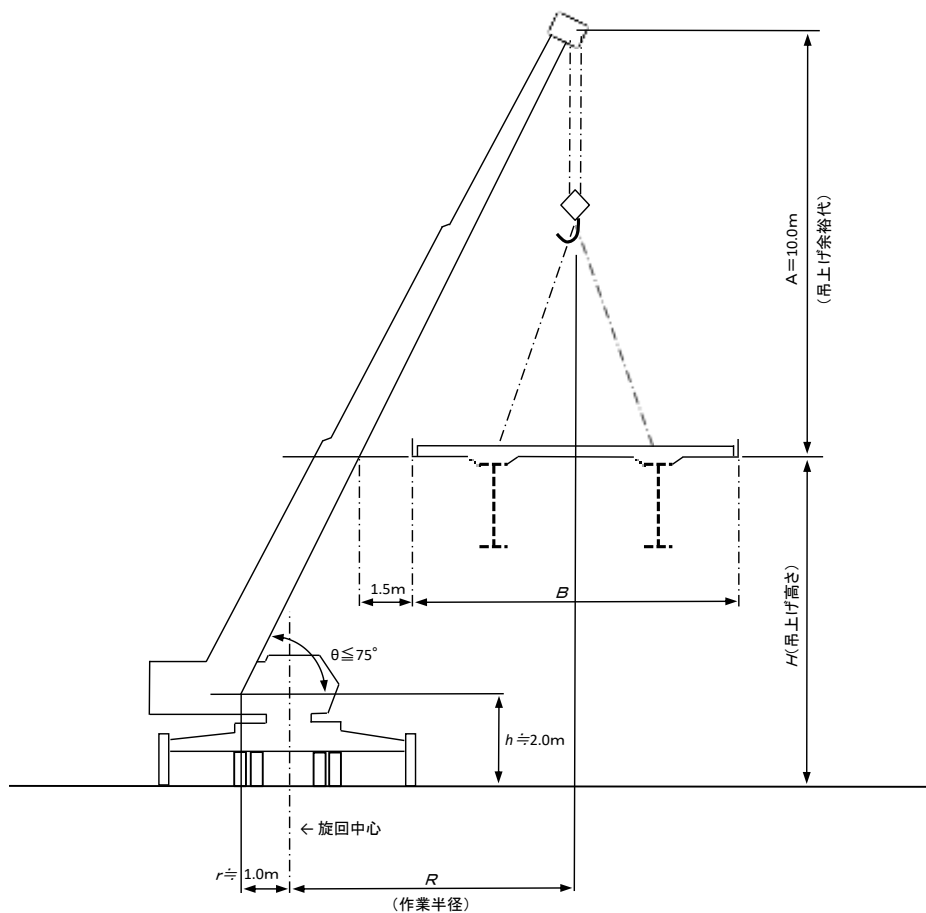
図 17.5 作業半径概略図・合成床版（トラッククレーン油圧伸縮ジブ型）
