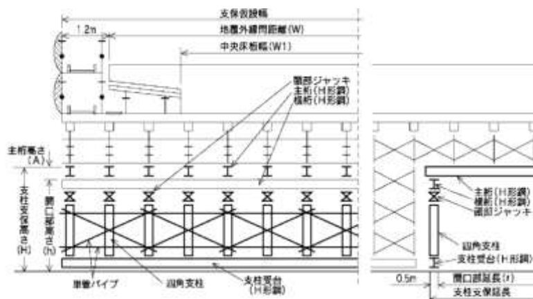
参考図 (支柱支保工概念図 (併用式))
