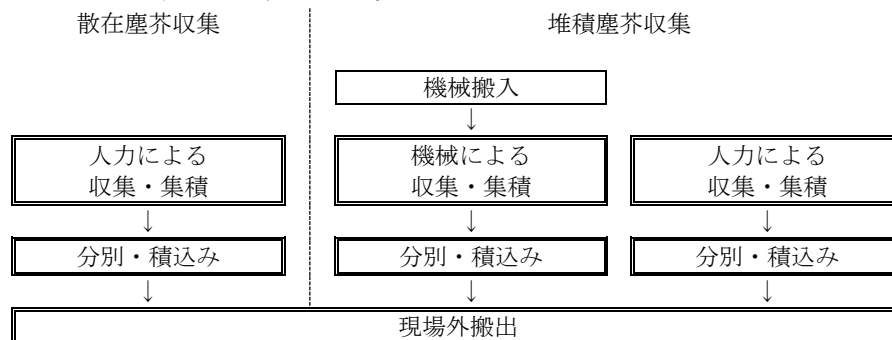
図 2-1 施工フロー
