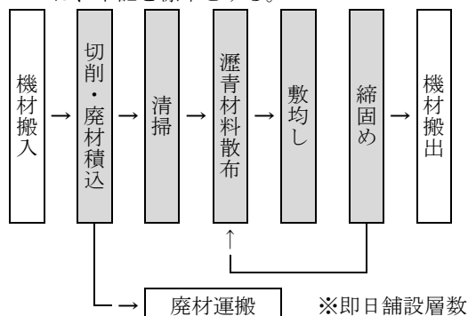
図 2.1 施工フロー
