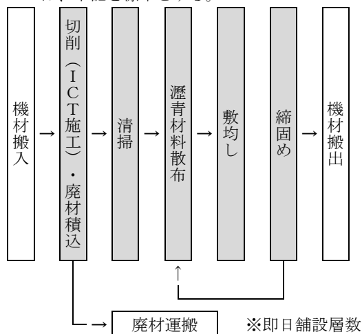
図 2.1 施工フロー
