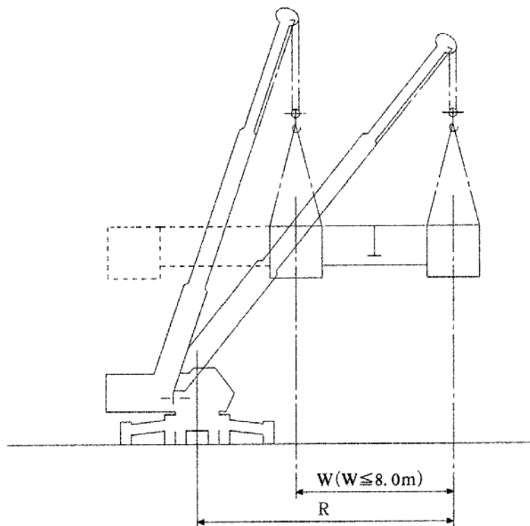
図 17.3 作業半径概略図・箱桁（トラッククレーン油圧伸縮ジブ型）
