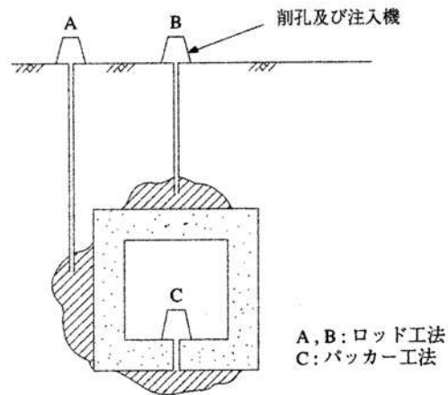
图 1-1 施工法
