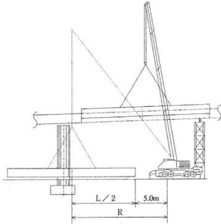
図 17.4 作業半径概略図（地組を伴う場合）
