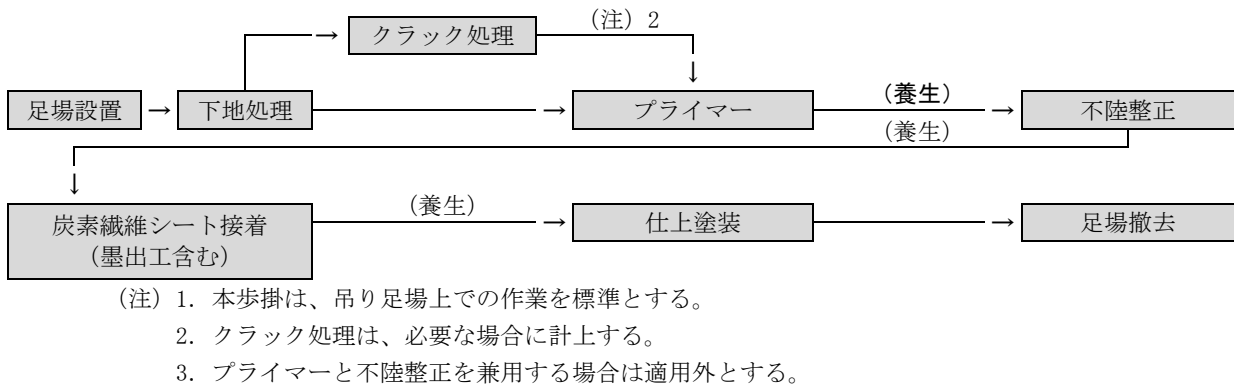
図 2-1 施工フロー
