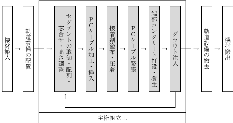
図 2-1 施工フロー
