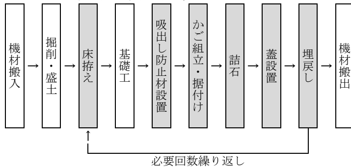
図 2-1 施工フロー
