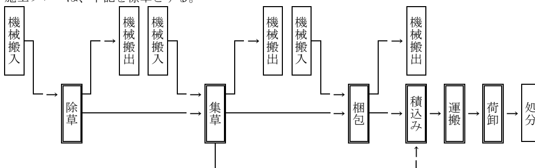
図 2-1 施工フロー
