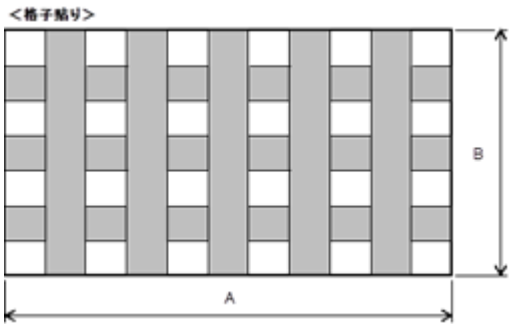
図 3.1 炭素繊維シート貼図 [参考図]
