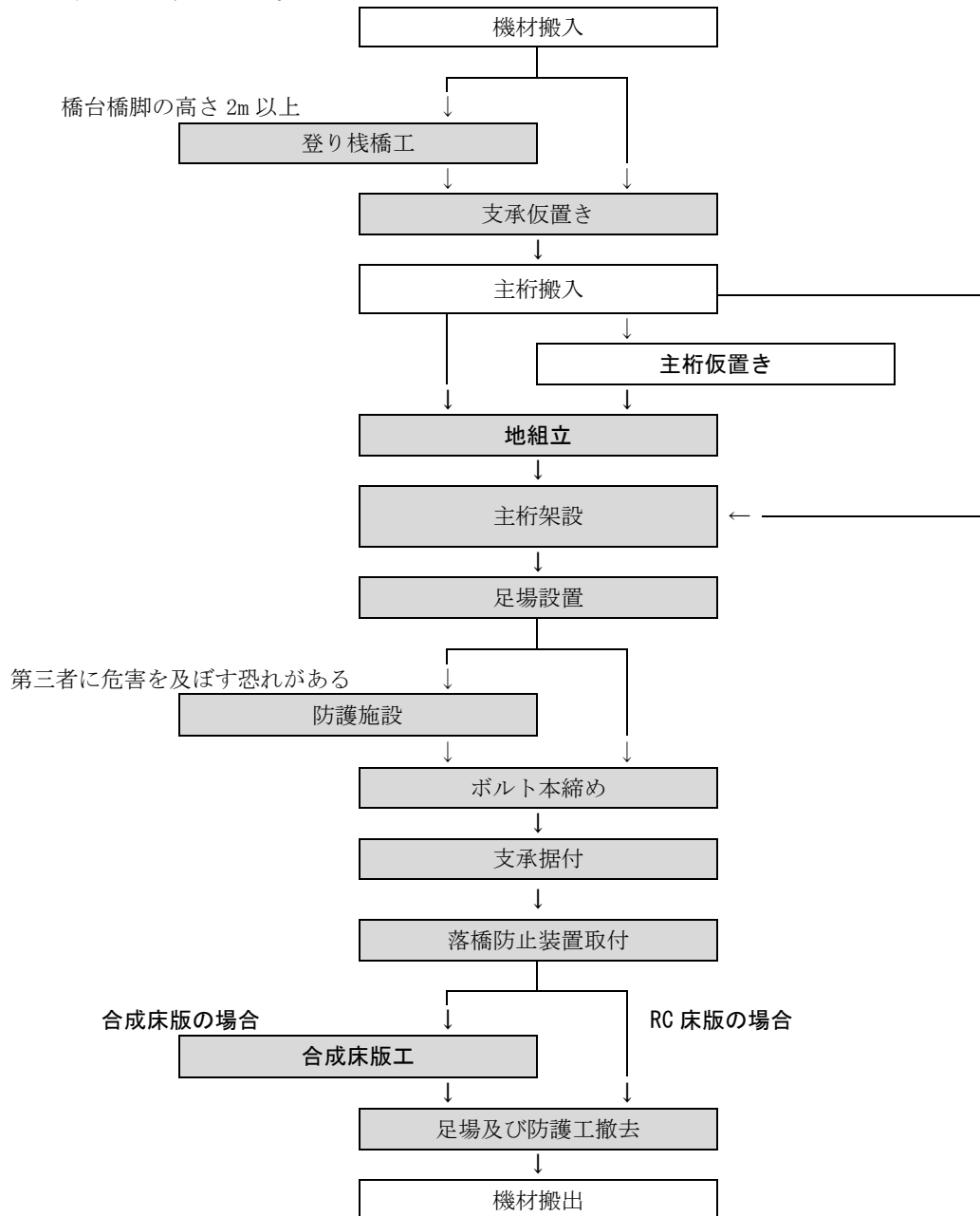
図 2-1 施工フロー
