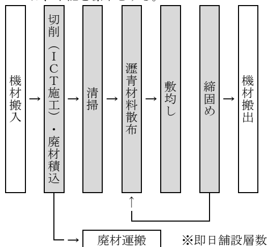
図 2.1 施工フロー
