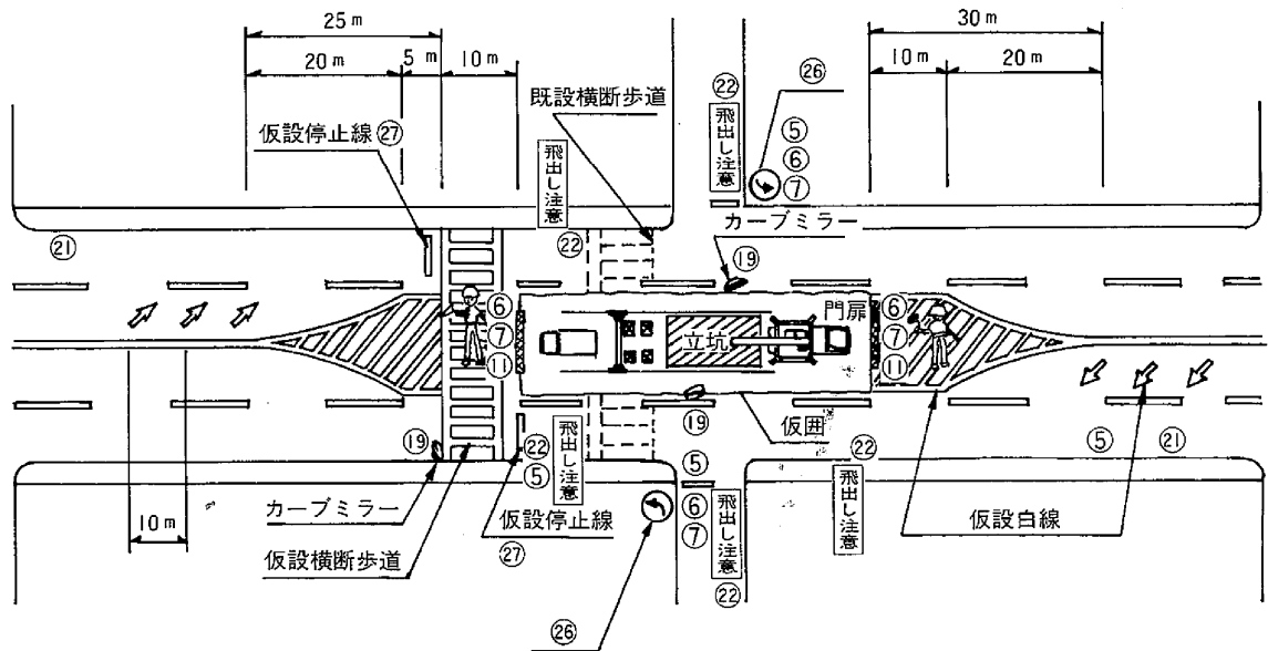
〔施工か所詳細図〕
