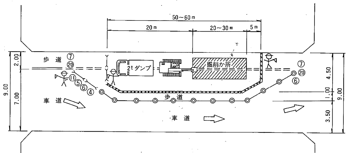
〔施工か所詳細図〕
