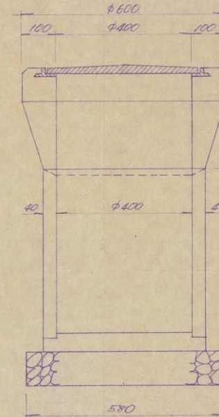
排水樹 (両型 2号) N:1/10
