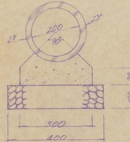
φ200ヒューム管敷設図 N:1/10
