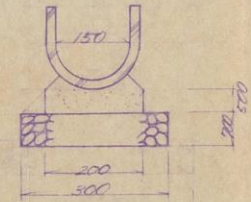
U型測溝敷設図 N:1/10
