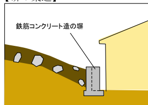
【塀の築造】
