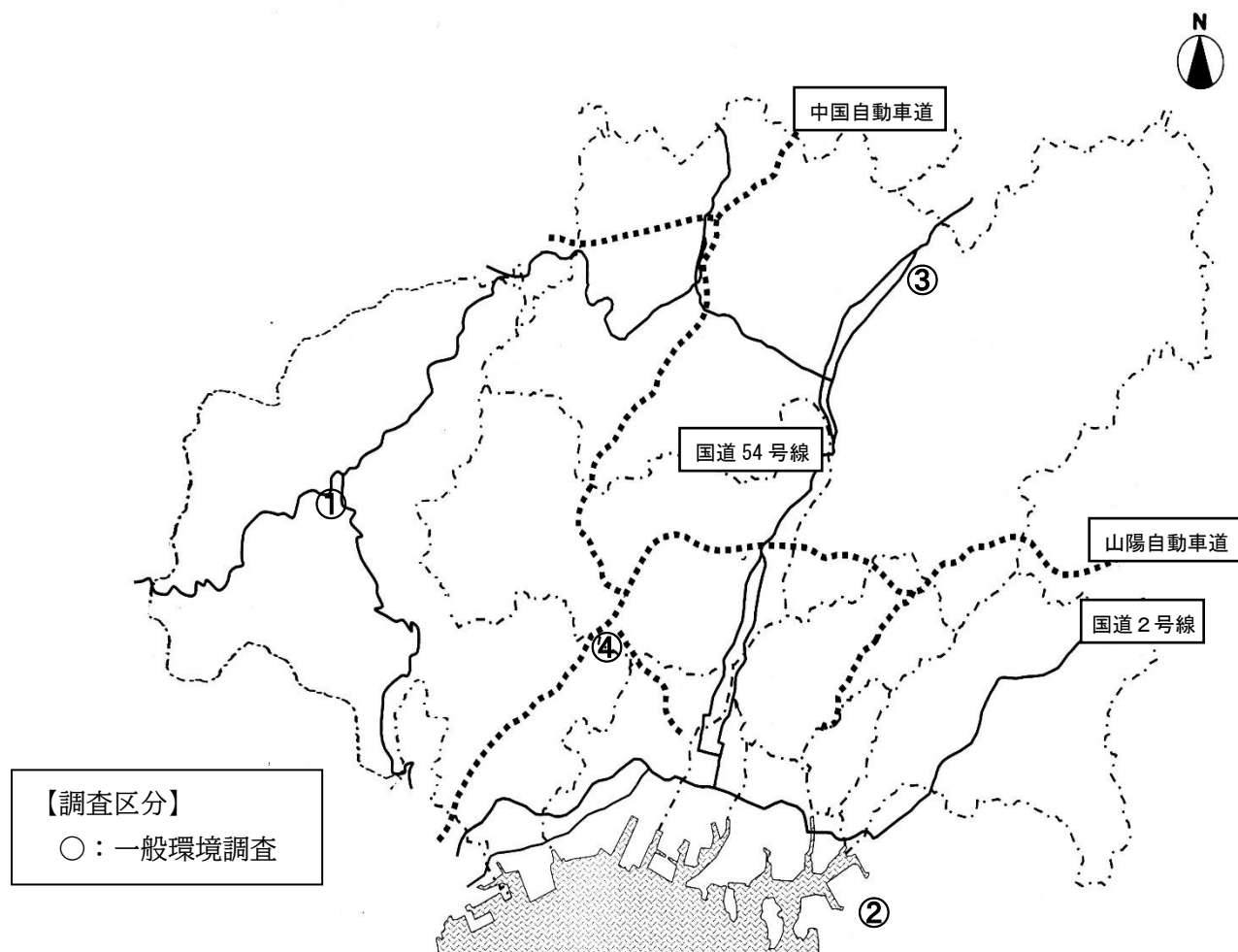
図26 大気測定車による測定地点図（令和5年度）
