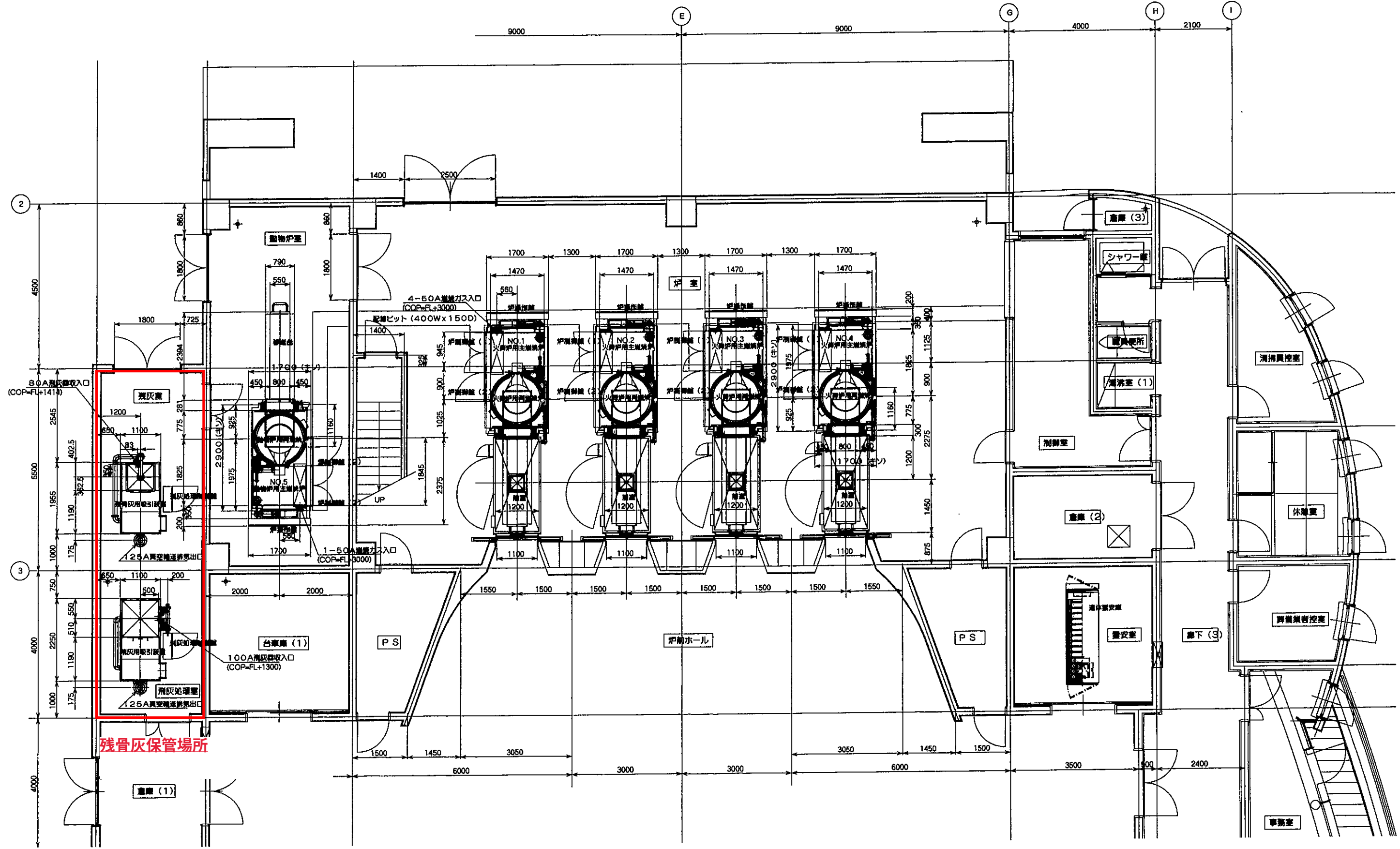
火葬炉1階平面配置図
