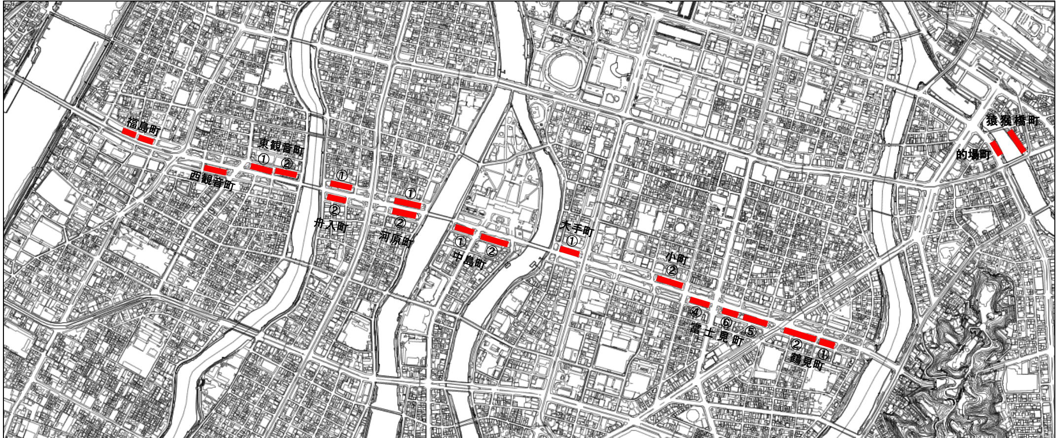
路上駐車場の施設位置図 (その他路外駐車場は個別位置図を参照)
