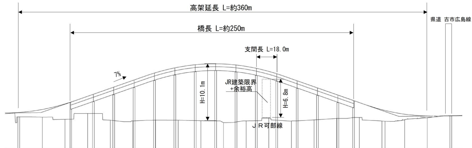
縦断図(高架部)
