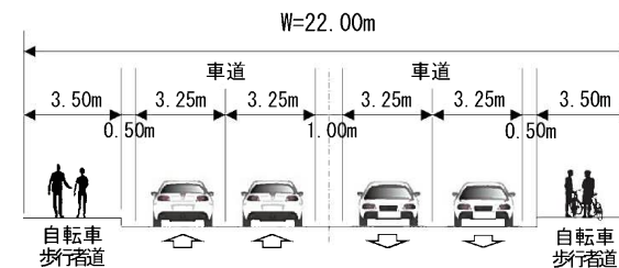
標準断面図（一般部）
