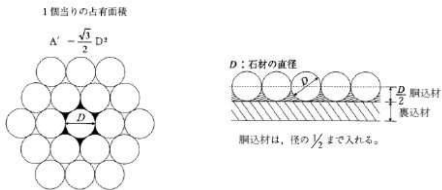
石材の基本数量表
