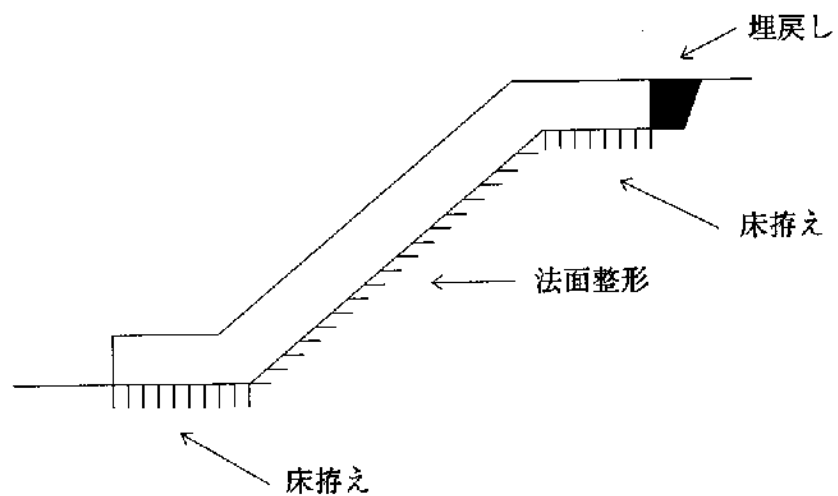
(2) ふとんかご (階段式)
