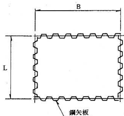
鋼矢板の場合
