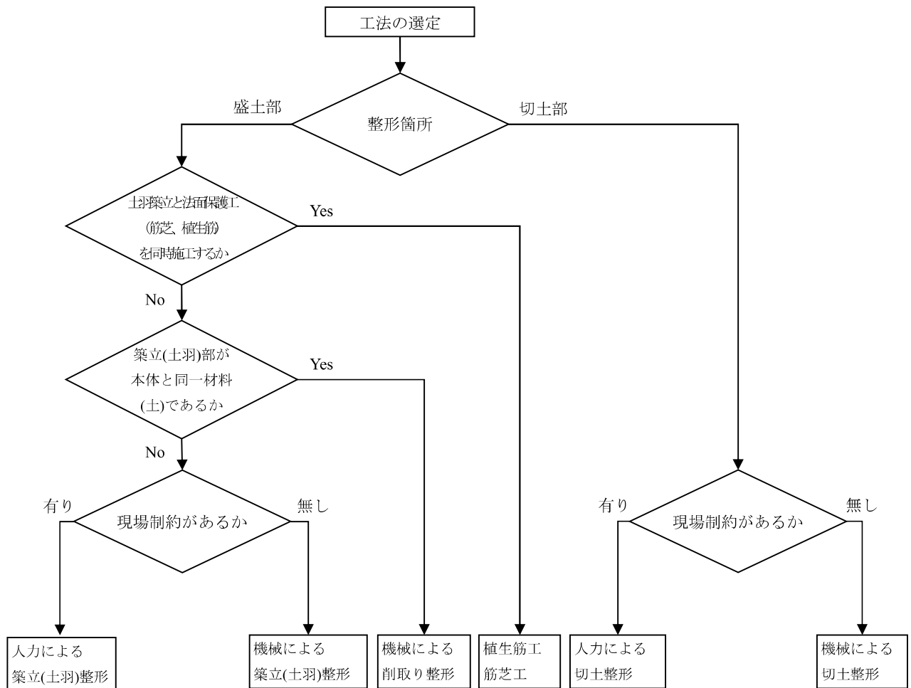
法面整形工 工法選定フロー図
