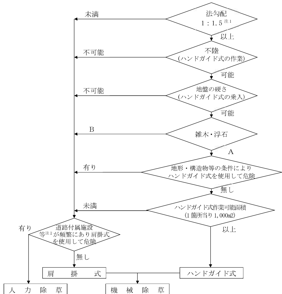
工法の選定フロー
