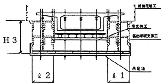
正面図
