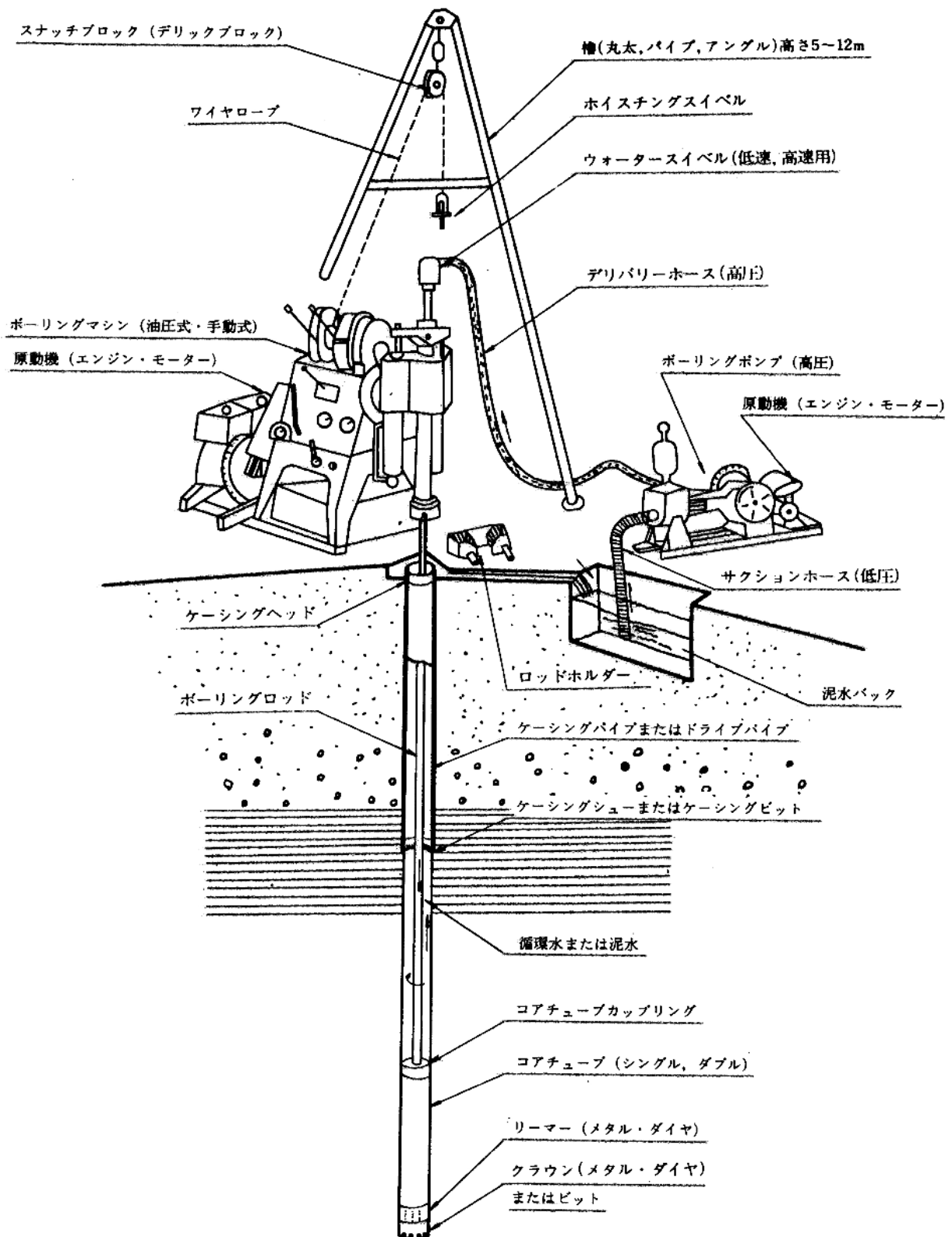
図 2-1-1 設備概念図
