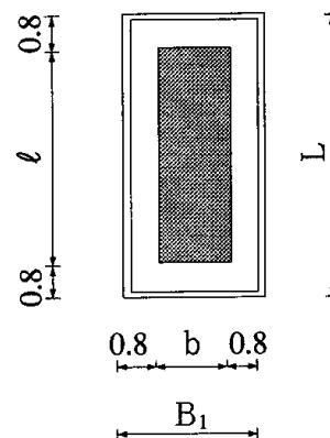
( 平 面 図 )
