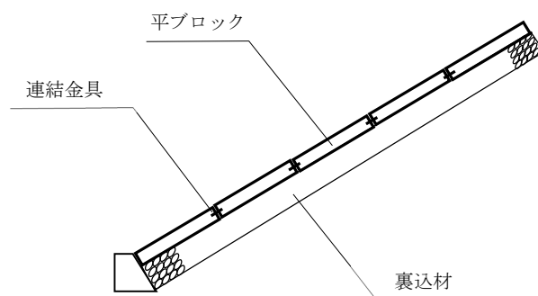
断面図
